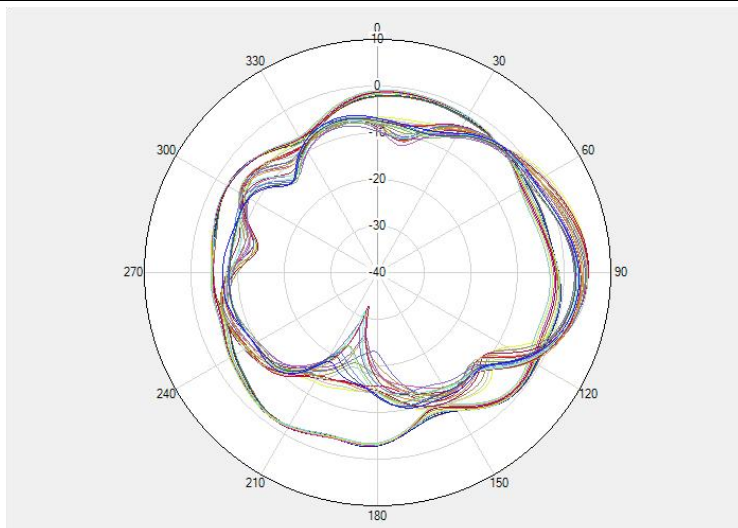
2400/5800MHZ-Phi 0
