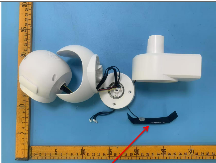
4G_ANT
