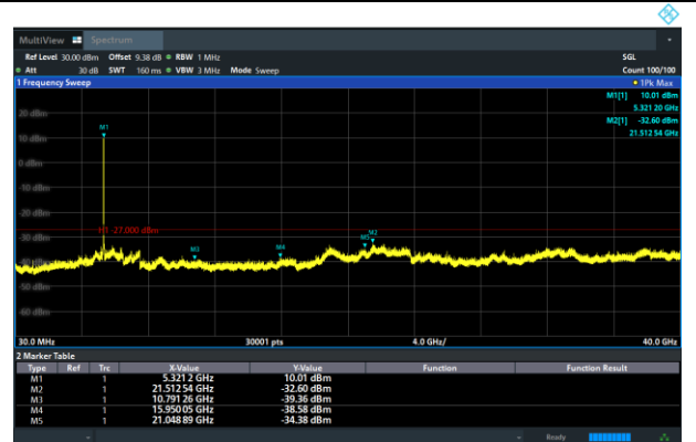
11ax (HE40) CH62
