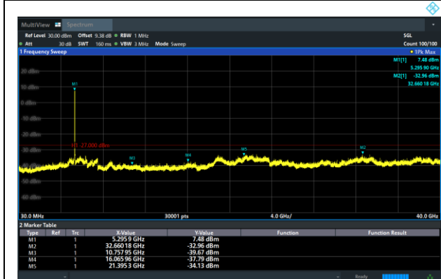
11ax (HE20) CH56
