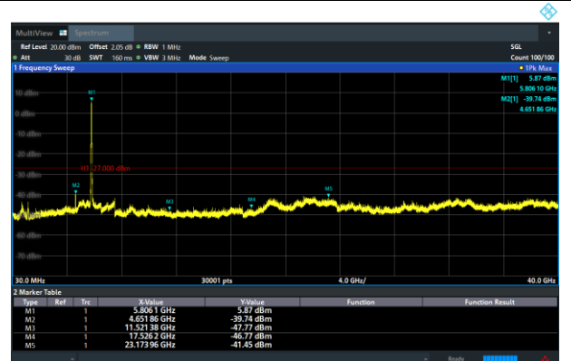
11ax(HE40) CH159
