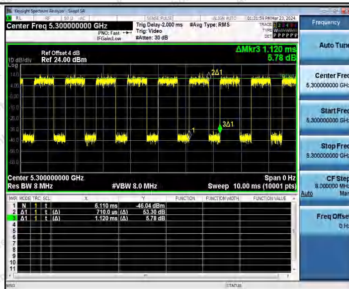
11A_Ant2_5300
