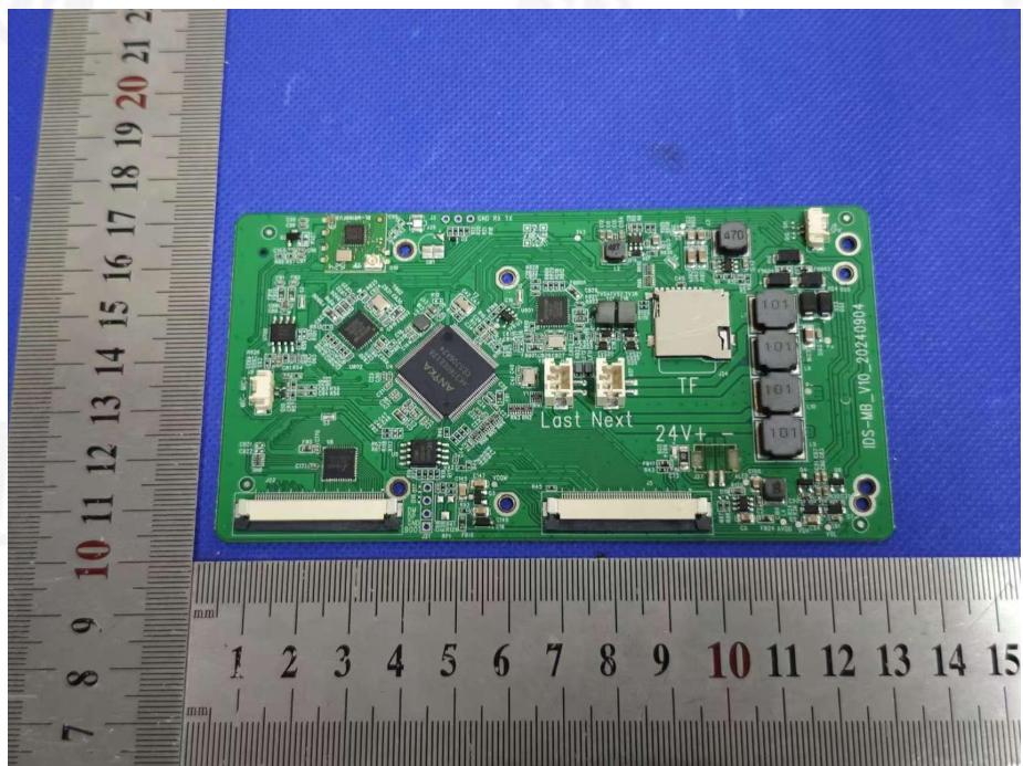
EUT Photo 3
