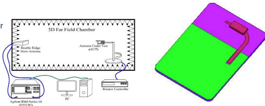
Fig.2 暗室示意图
