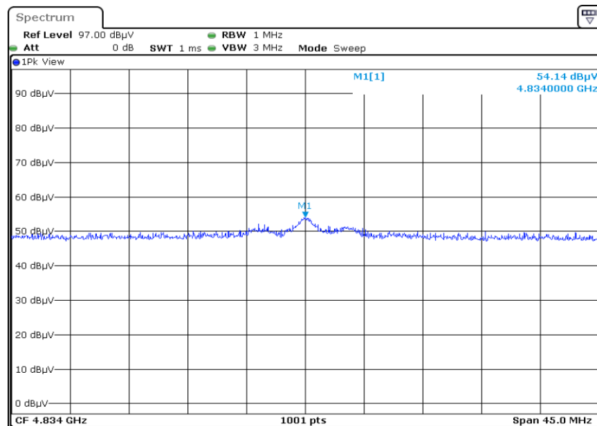
F1 X2 4834.0 Harmonic Horizontal PEAK
