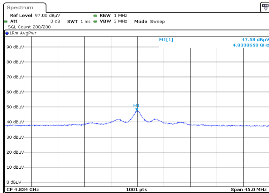
F1 X2 4834.0 Harmonic Horizontal AVG
