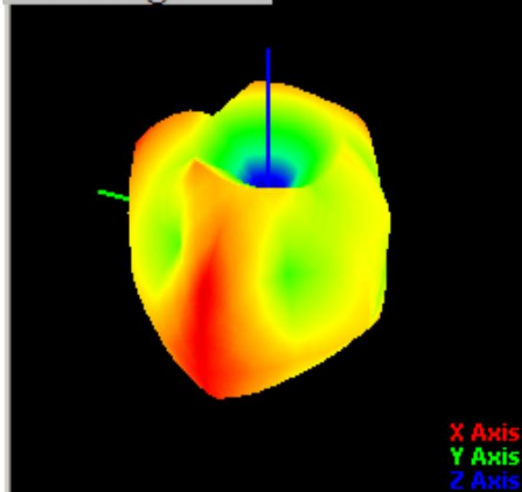
5275.00MHz@T45P200
