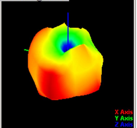
5350.00MHz@T45P200
