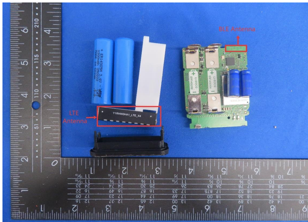
(10) EUT Photo
