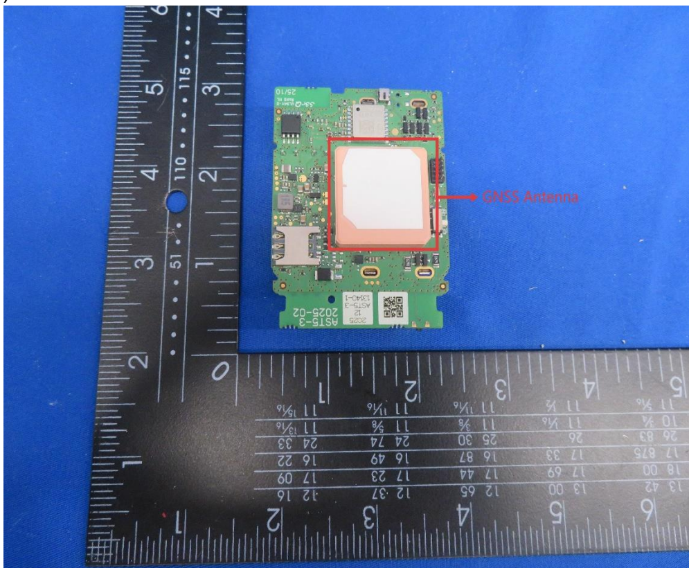
(14) EUT Photo
