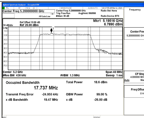
11AC20MIMO-Ant1-5200
