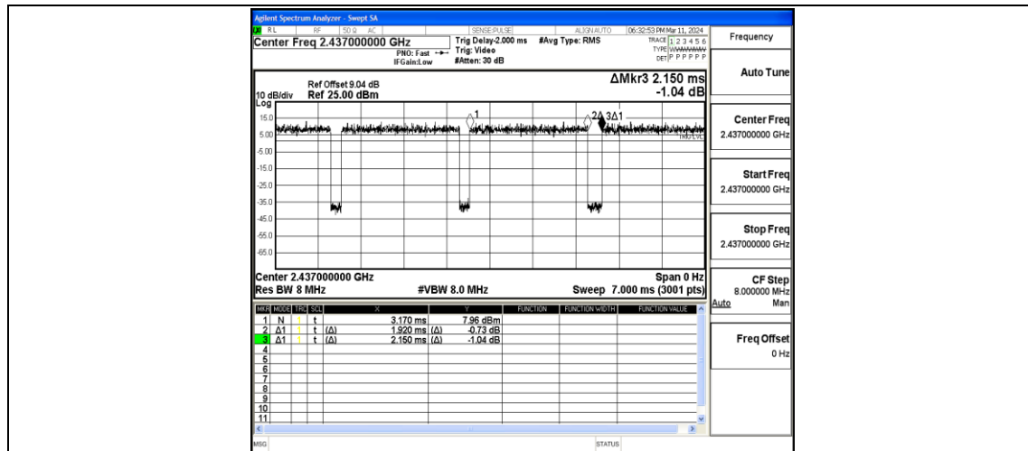
NTNV-11N20MIMO-Ant2-2437
