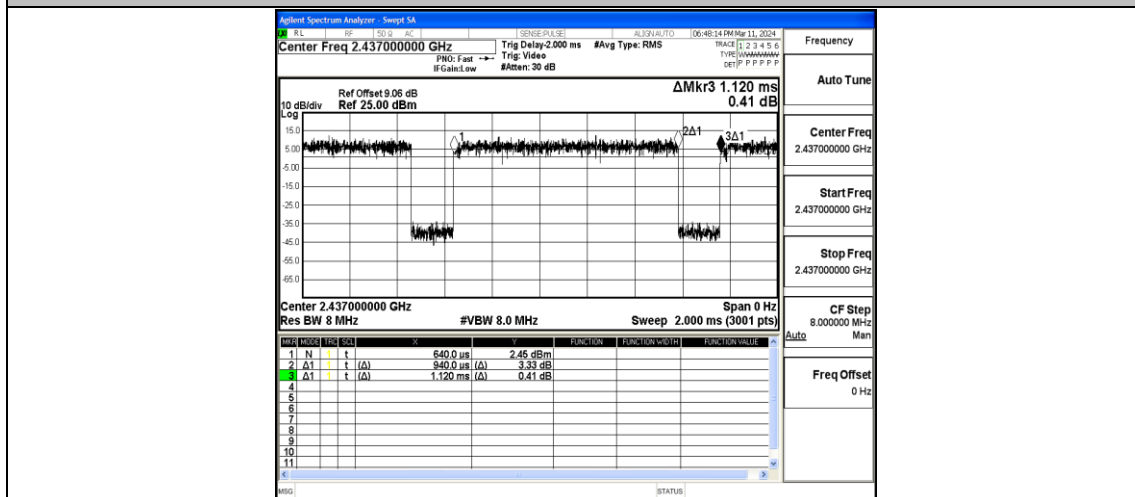
NTNV-11N40MIMO-Ant1-2437
