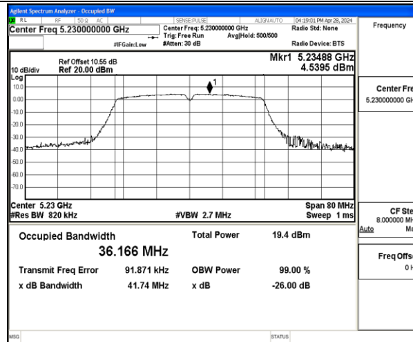
11AC40MIMO-Ant1-5230
