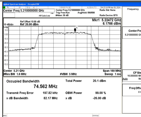
11AC80MIMO-Ant1-5210
