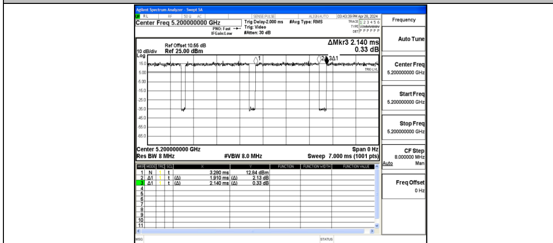
NTNV-11N20MIMO-Ant1-5200
