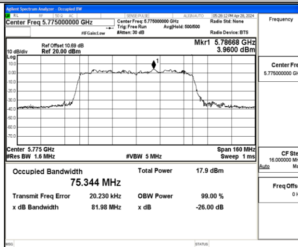
11AC80MIMO-Ant1-5775
