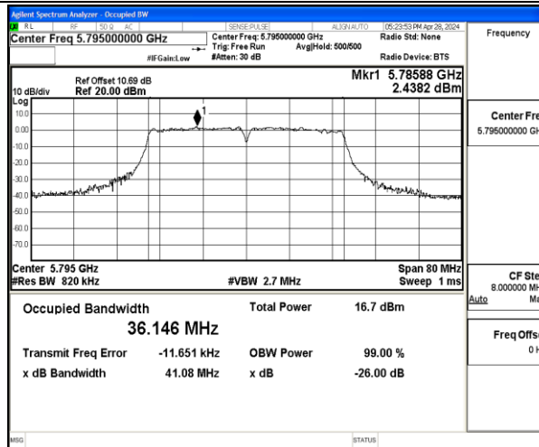
11AC40MIMO-Ant1-5795
