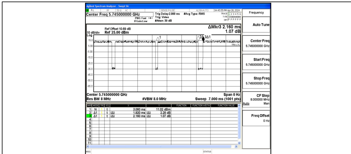
NTNV-11N20MIMO-Ant1-5745
