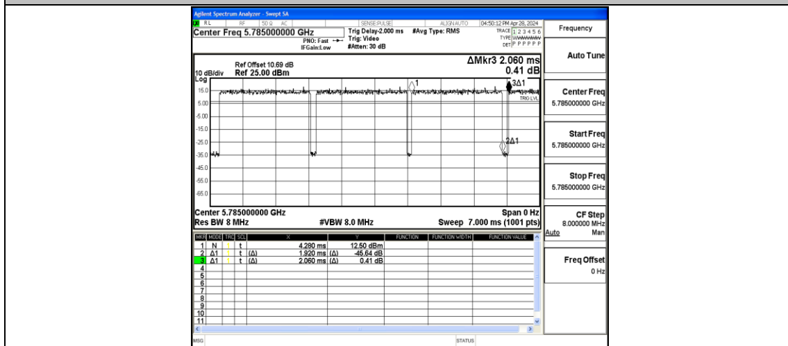
NTNV-11N20MIMO-Ant1-5785
