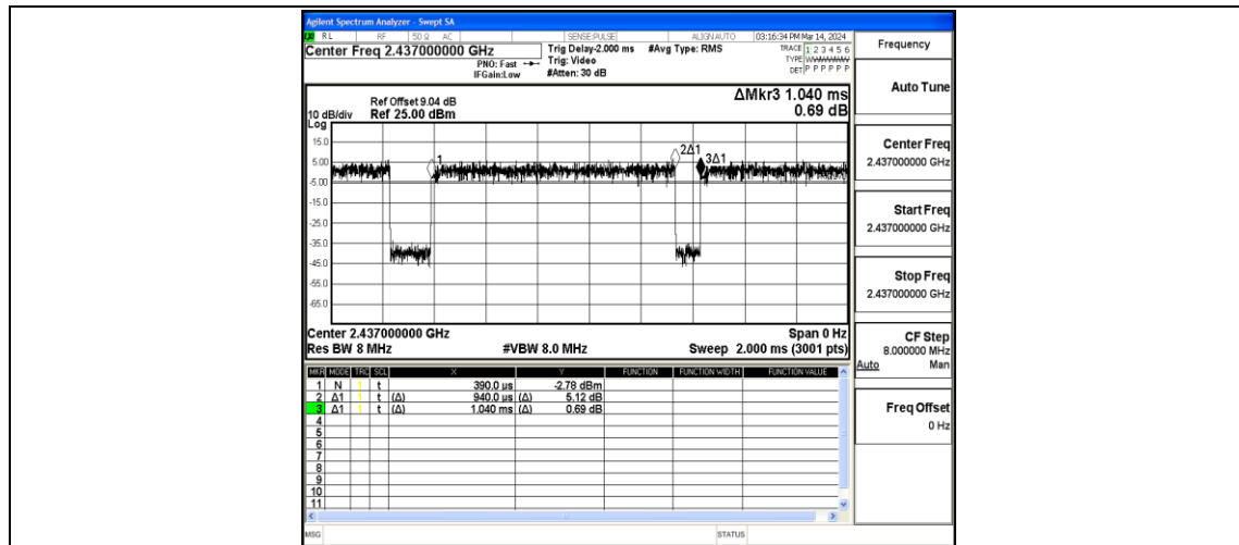
NTNV-11N40MIMO-Ant2-2437
