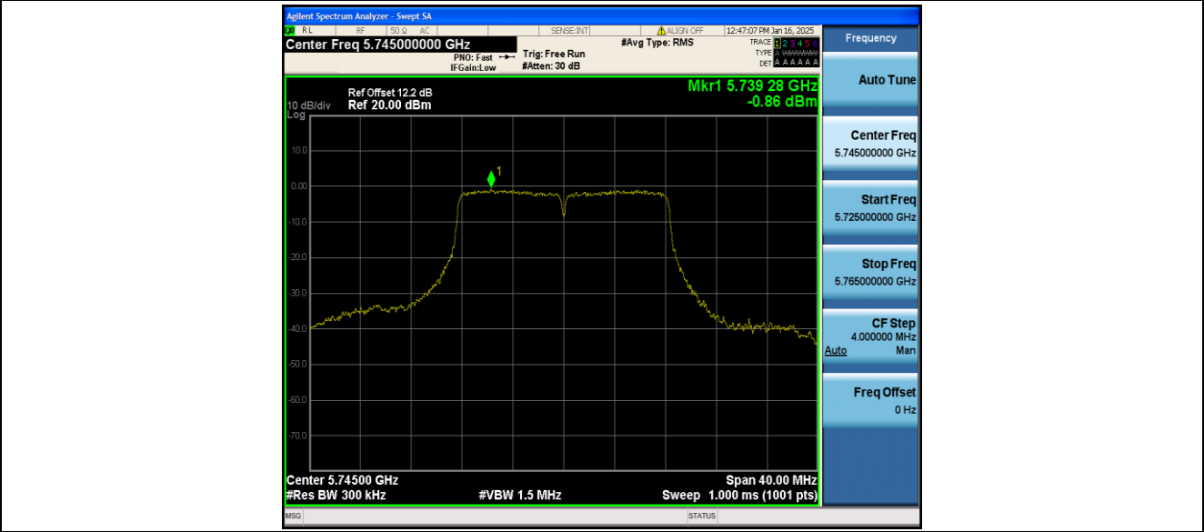
11A_Ant2_5745
