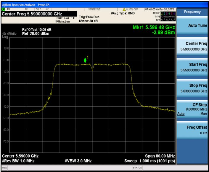
11N40MIMO_Ant2_5590
