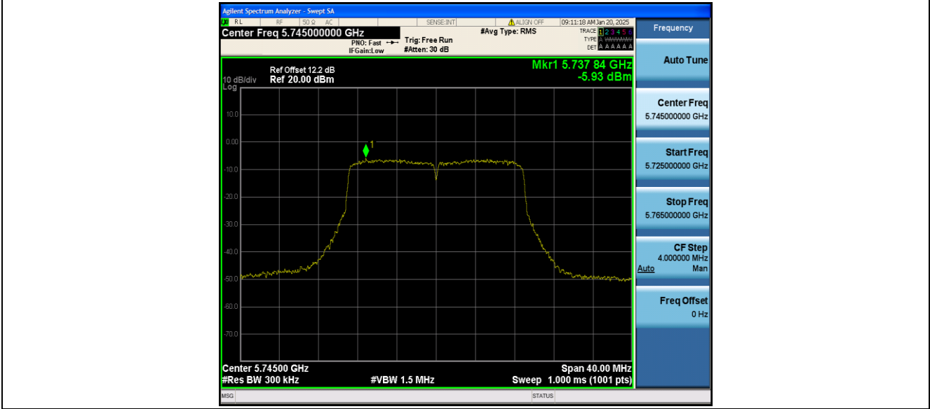
11AC20MIMO_Ant1_5745
