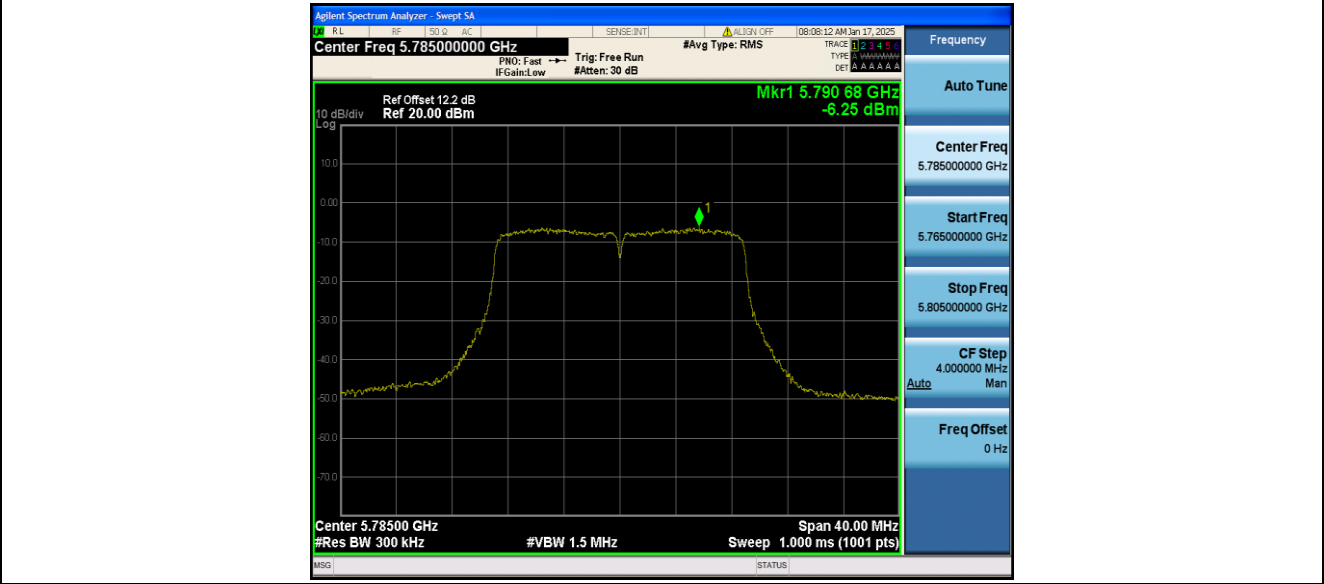
11N20MIMO_Ant1_5785
