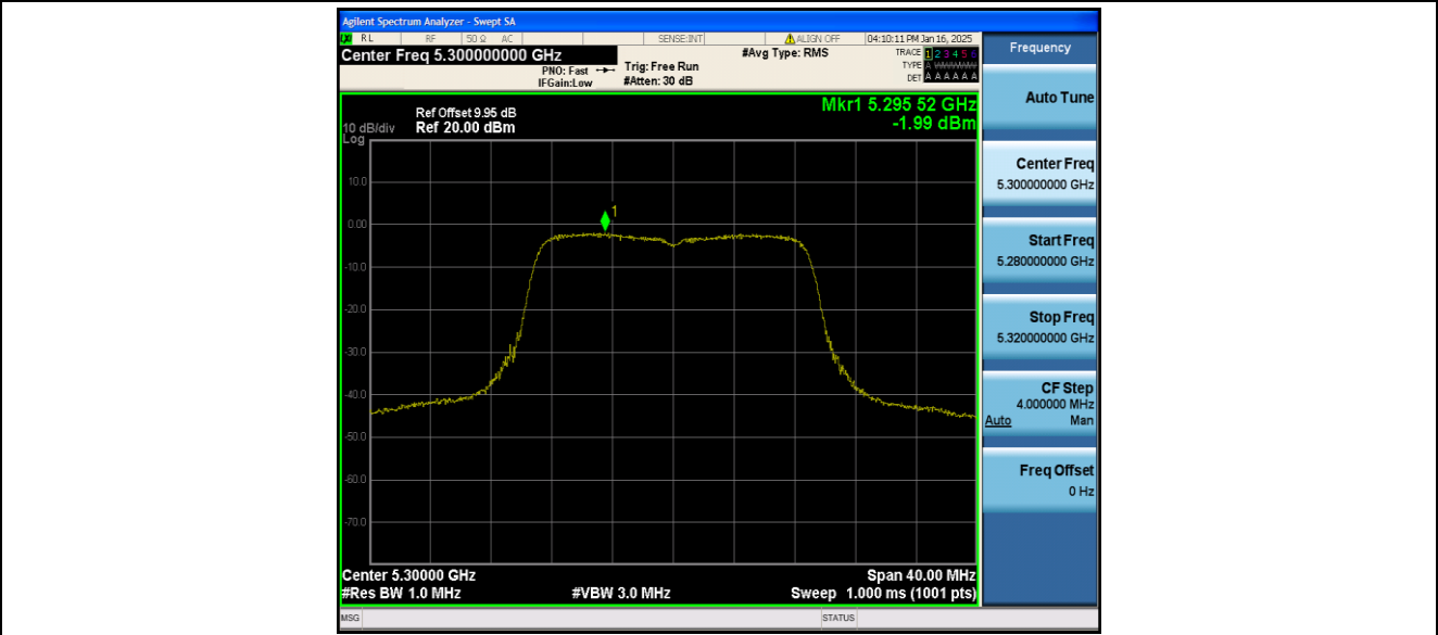
11N20MIMO_Ant2_5300
