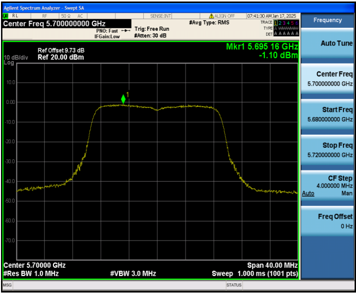
11N20MIMO_Ant2_5700
