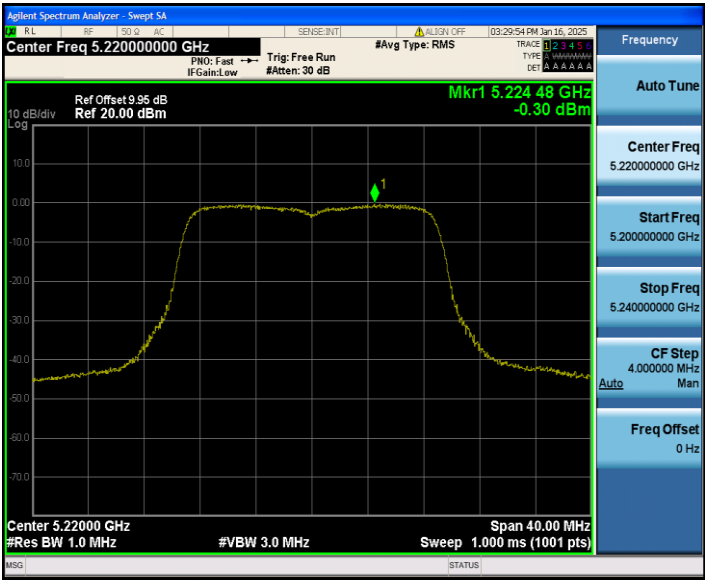
11N20MIMO_Ant2_5220
