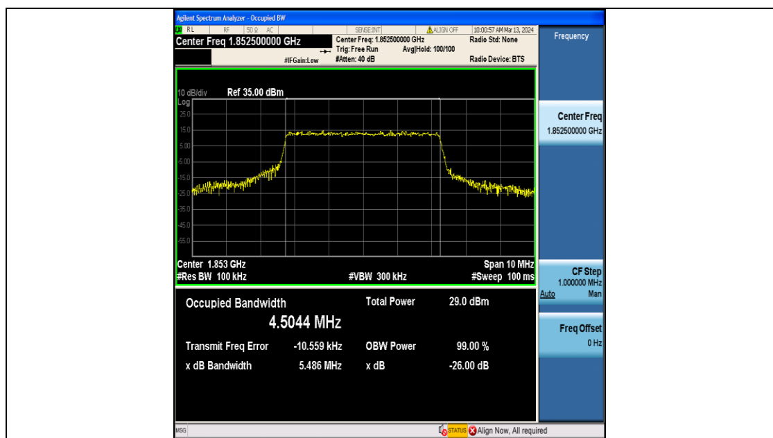
Band2-5MHz-QPSK-18625-25RB#0-PASS
