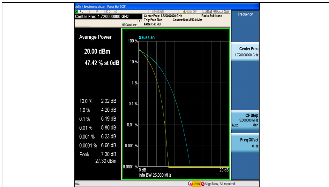
Band4-20MHz-QPSK-20050-100RB#0-PASS
