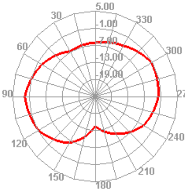
2400.000MHz E2
