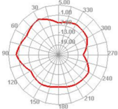
2500.000MHz H
