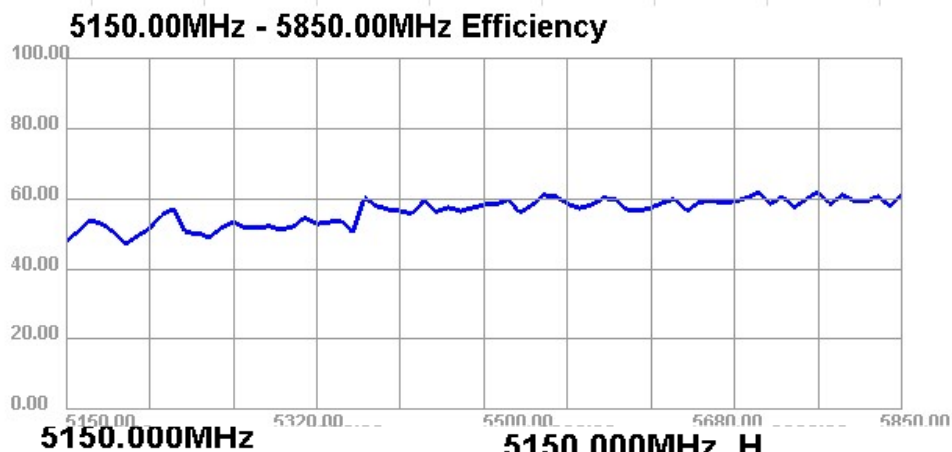
5150.000MHz H
