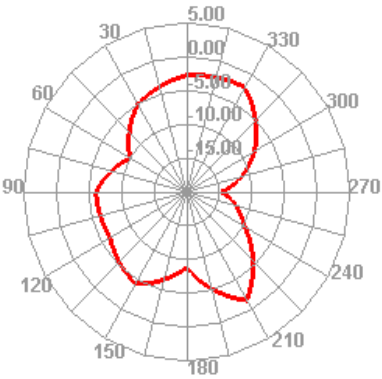
2400.000MHz E1
