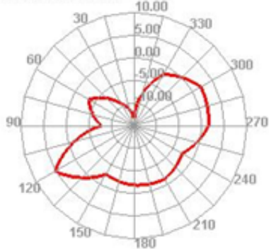
5850.000MHz E1
