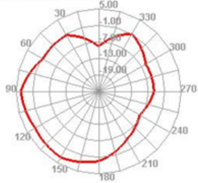
5500.000MHz E2
