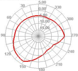
2400.000MHz E2
