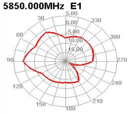
5850.000MHz E1
