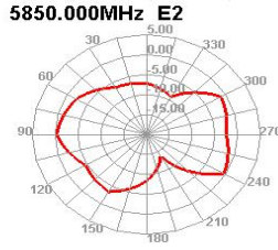
5850.000MHz E2
