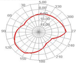
2450.000MHz E2
