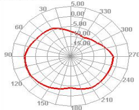
2500.000MHz E1
