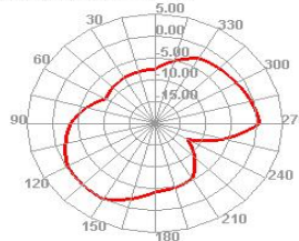
2500.000MHz E2
