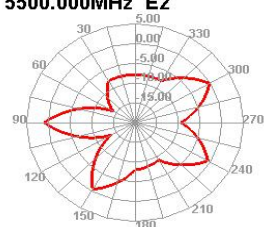
5500.000MHz E2
