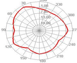
2450.000MHz H
