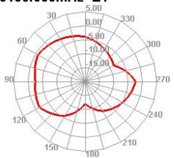
5150.000MHz E1
