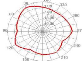
2500.000MHz E2
