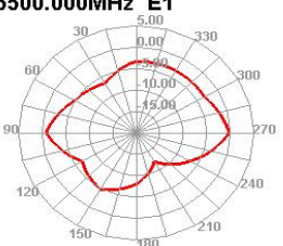
5500.000MHz E1
