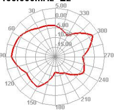
5150.000MHz E2
