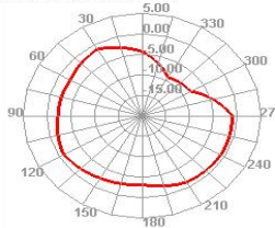
2450.000MHz E1
