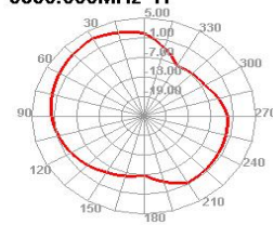
5850.000MHz H
