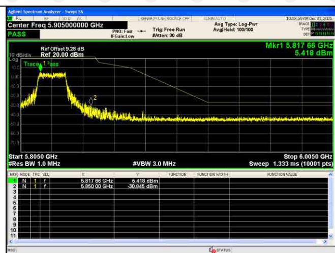
802.11(n40)-5795
