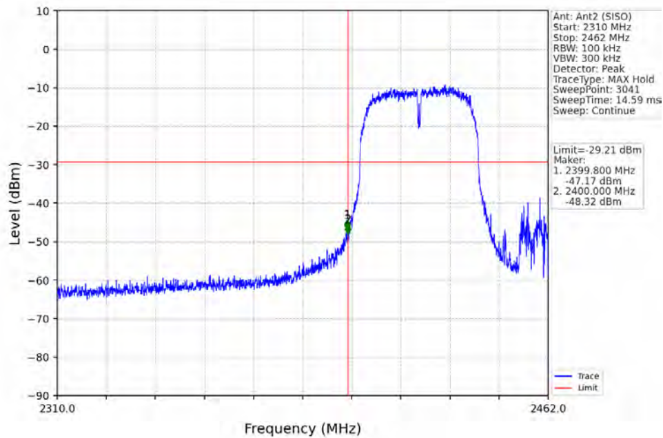
802.11n(HT40)_LCH_2422MHz_Ant2 (SISO)_NTNV
