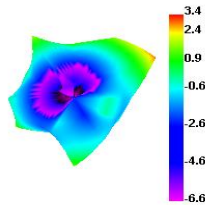
2450.000MHz E1
