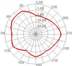
2400.000MHz E2
