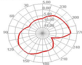
2500.000MHz E2
