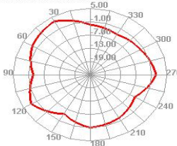
2450.000MHz H
