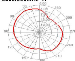
5850.000MHz H
