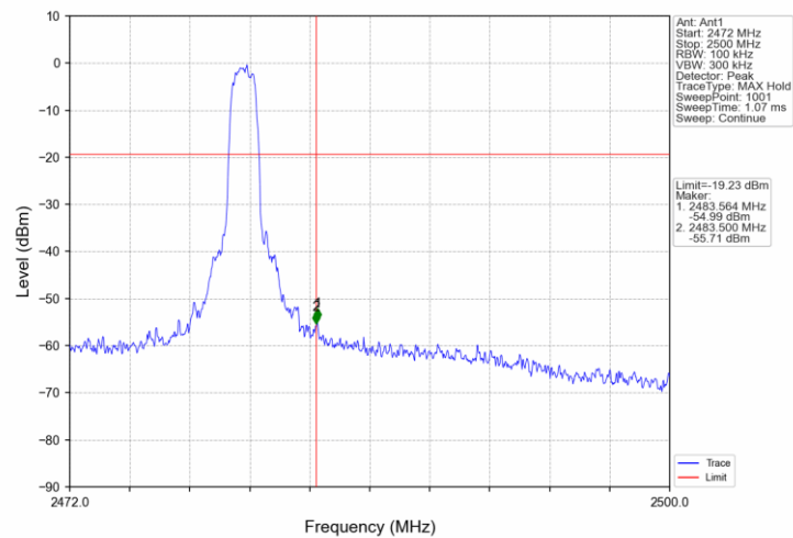
8DPSK 3DH5_HOPP_Ant1_NTNV
