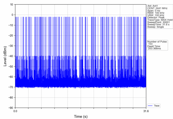
Pi/4DQPSK_2DH5_HOPP_Ant1_NTNV
