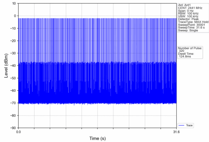
8DPSK 3DH3_HOPP_Ant1_NTNV
