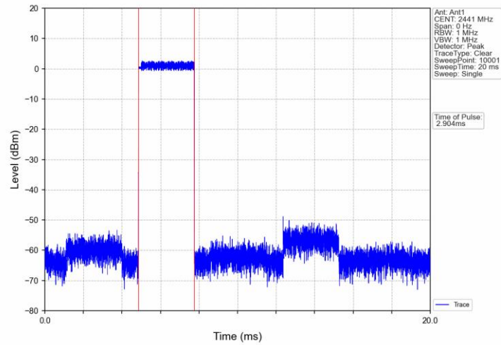
Pi/4DQPSK 2DH5 HOPP Ant1 NTN
