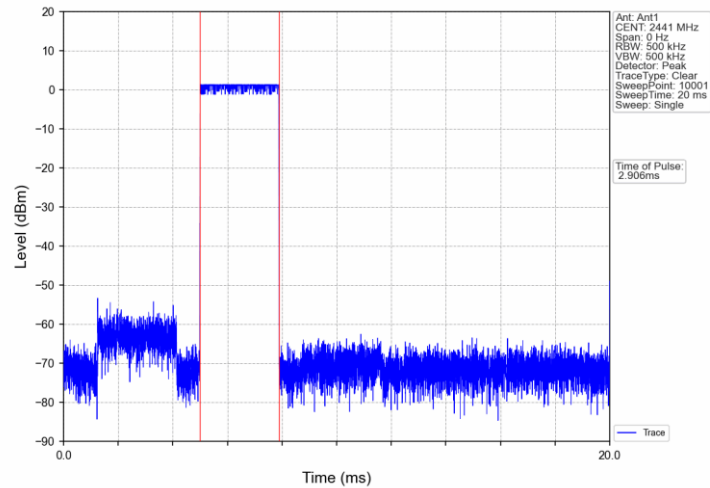
GFSK DH5 HOPP Ant1 NTNv
