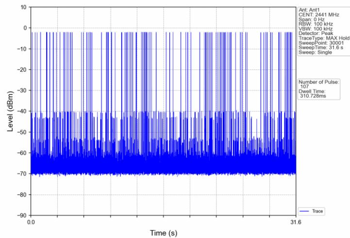
8DPSK 3DH1 HOPP Ant1 NTN
