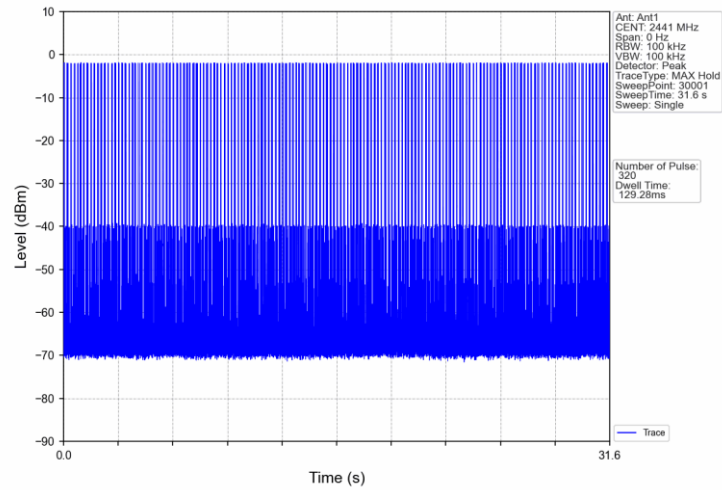
Pi/4DQPSK_2DH3_HOPP_Ant1_NTNV
