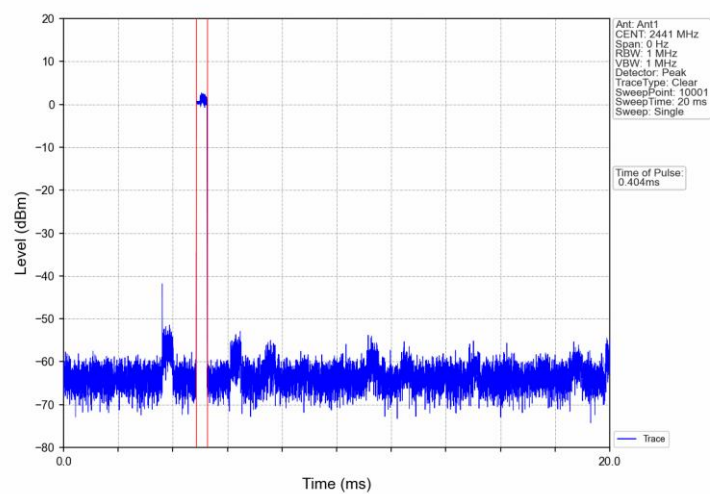
Pi/4DQPSK 2DH1 HOPP Ant1 NTNv
