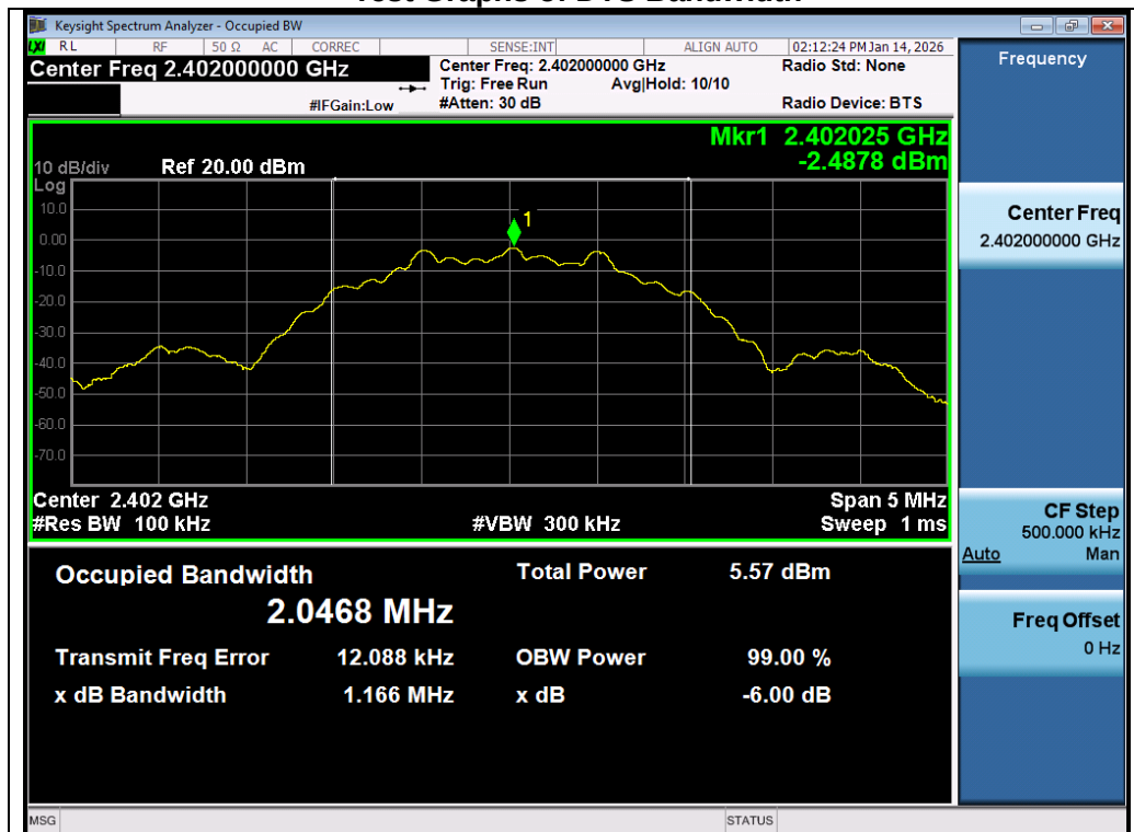
Test_Graph_2.4G_ANT1_2402_GFSK_DTSBW
