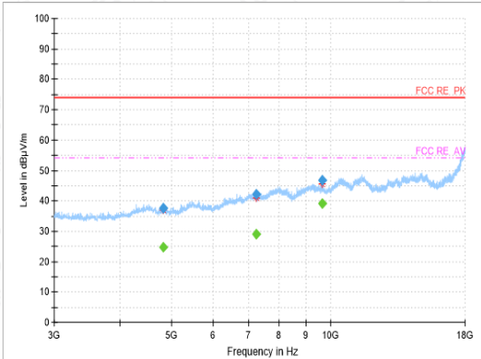
RSE-11N(20M)-CH1-3GHz-18GHz
