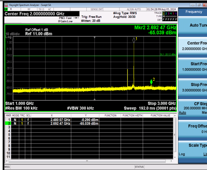
BLE_125K_Ant1_2480_3000~5000
