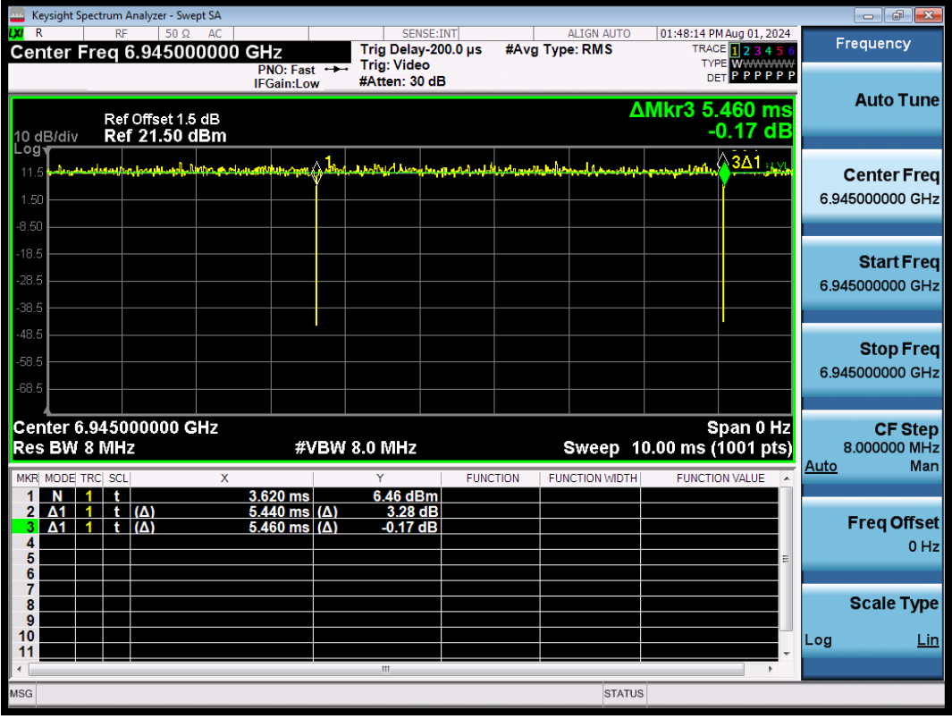
NTNV-11AX80SISO-Ant1-6945
