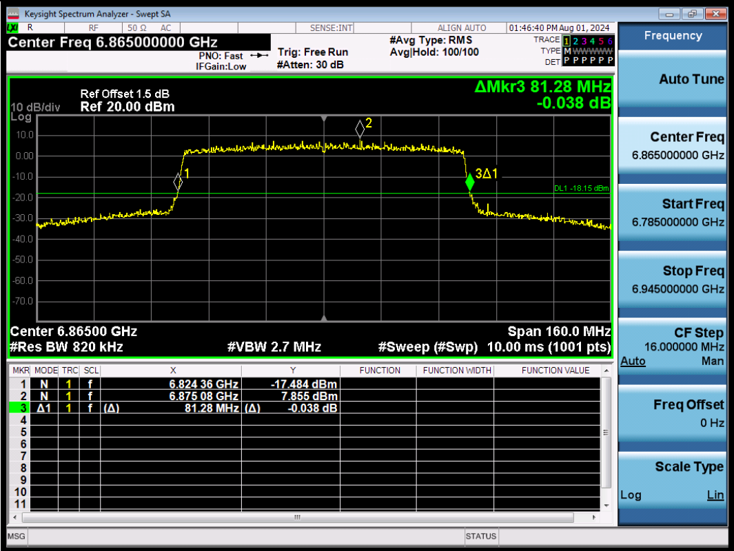
11AX80SISO-Ant1-6865
