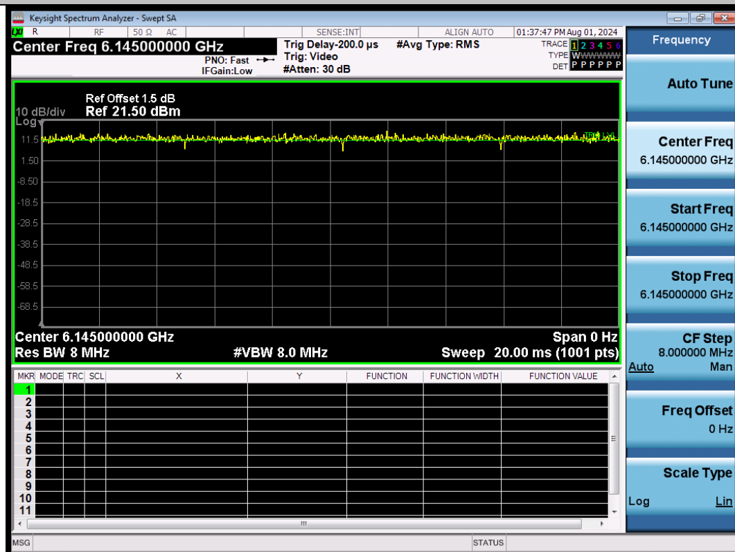
NTNV-11AX80SISO-Ant1-6145
