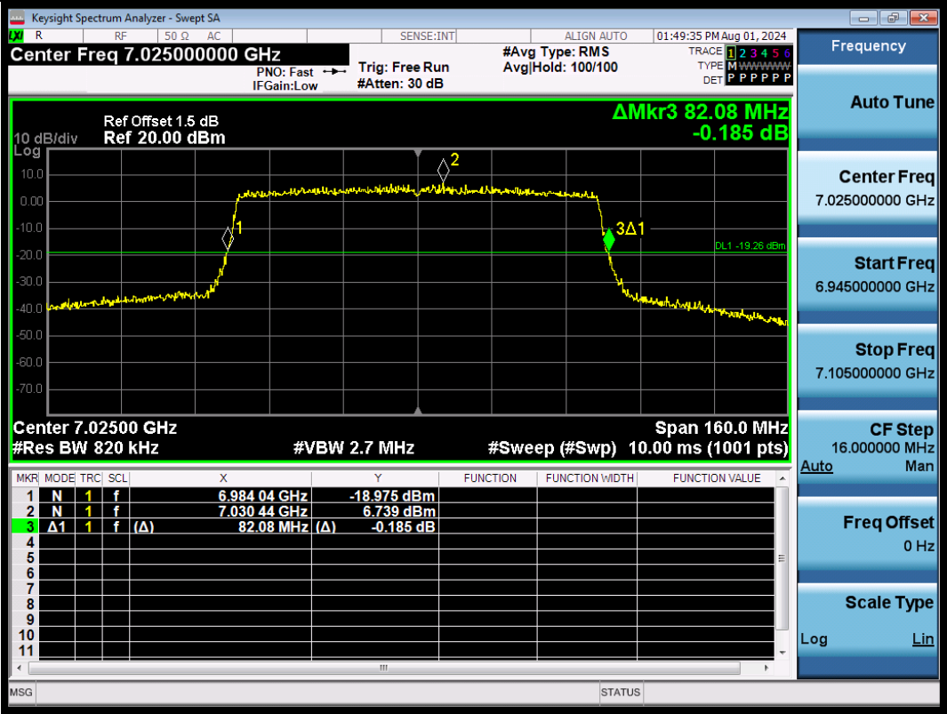
11AX80SISO-Ant1-7025
