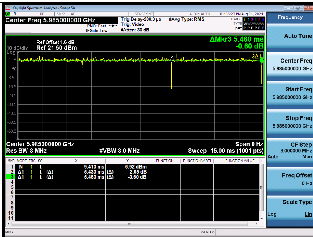
NTNV-11AX80SISO-Ant1-5985
