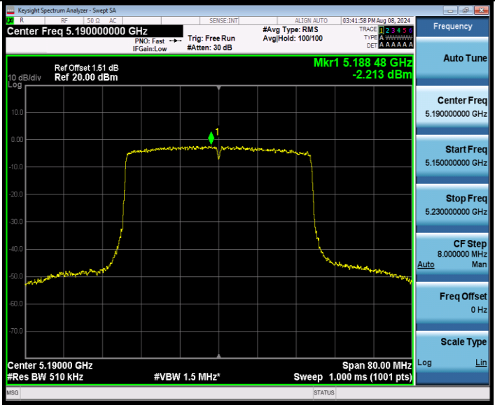
11AX40SISO_Ant1_5230
