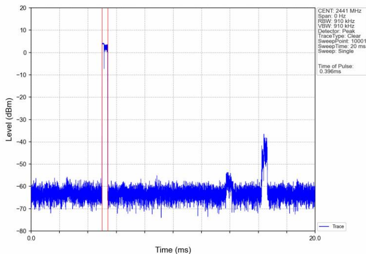
8DPSK_3DH1_HOPP_Ant1_NTNV
