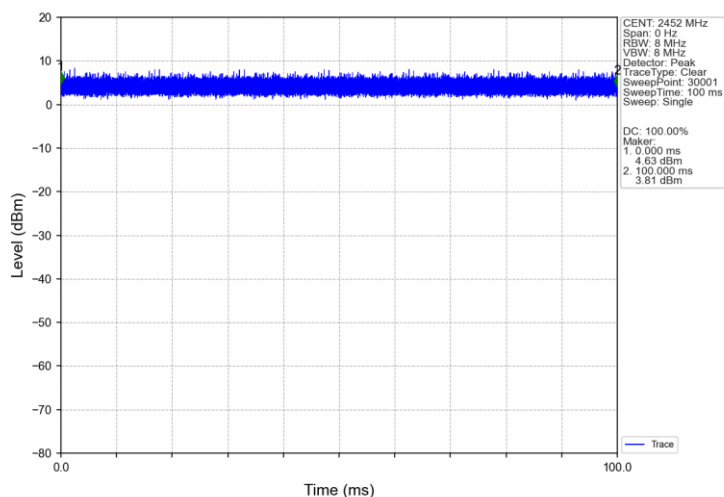
802.11n(HT40)_HCH_2452MHz_Ant1 (SISO)_NTNV
