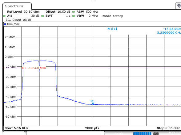
802.11n40_5190MHz
