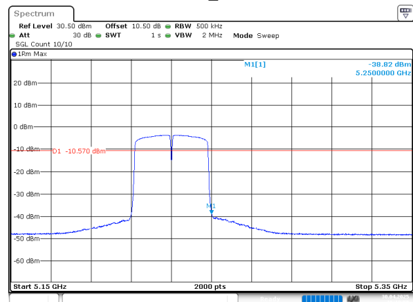
802.11n40_5230MHz
