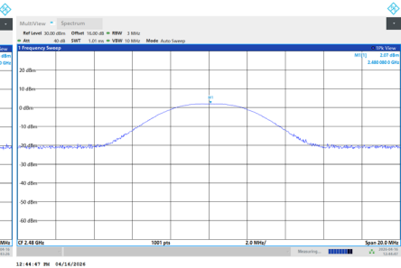
CH39
