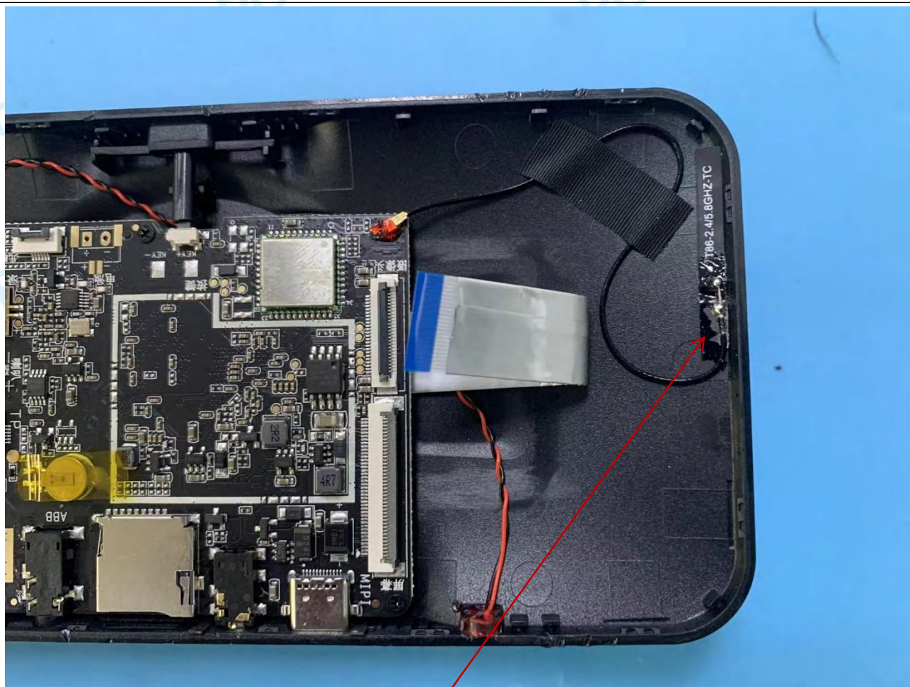
BLE-ANT
