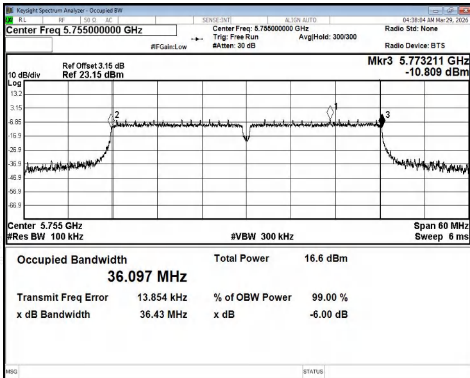
-6dB Bandwidth NVNT ac40 5755MHz Ant1
