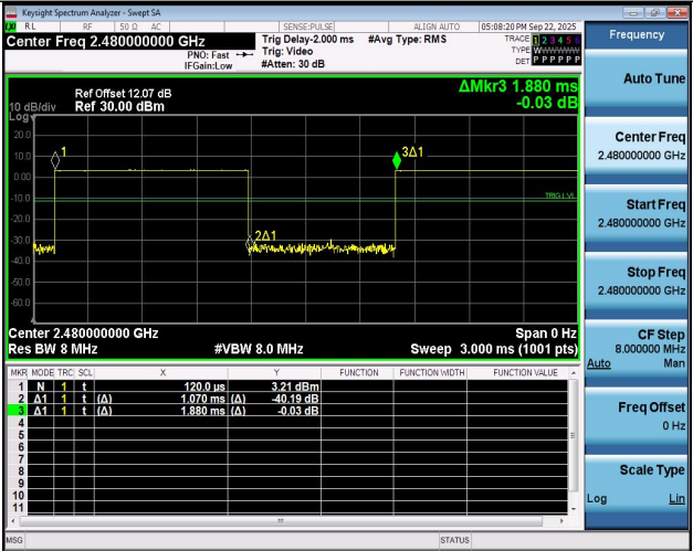
NTNV-LE_2M-Ant1-2480
