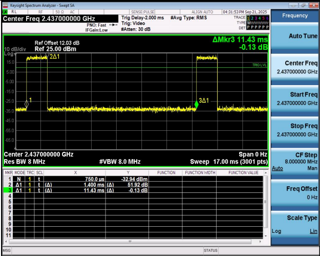
NTNV-11G-Ant1-2437
