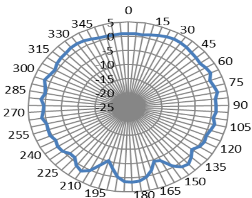
YZ-2450MHz
