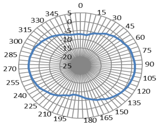
XY-2450MHz
