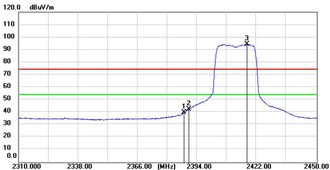
11n(HT20)_TX_CH_01_Vertical_Average
