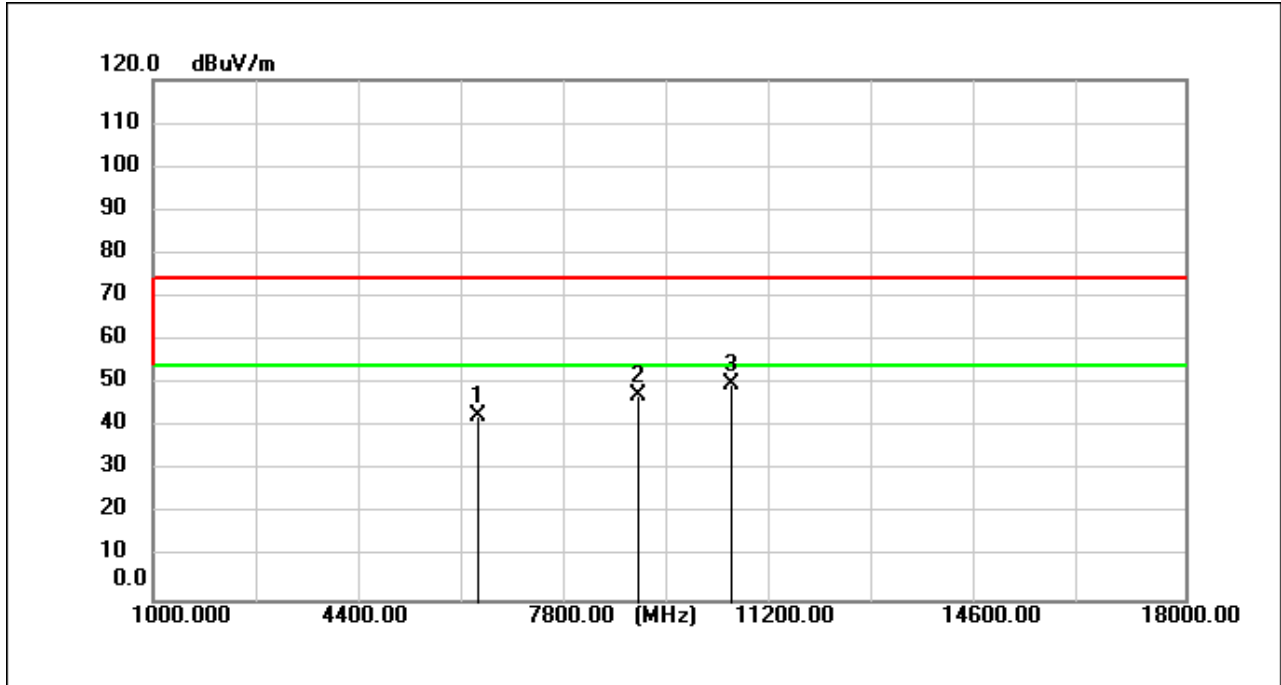
11b_TX_CH_01_Horizontal
