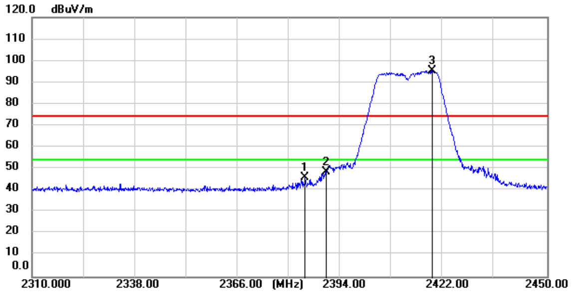
11n(HT20)_TX_CH_01_Horizontal_Peak
