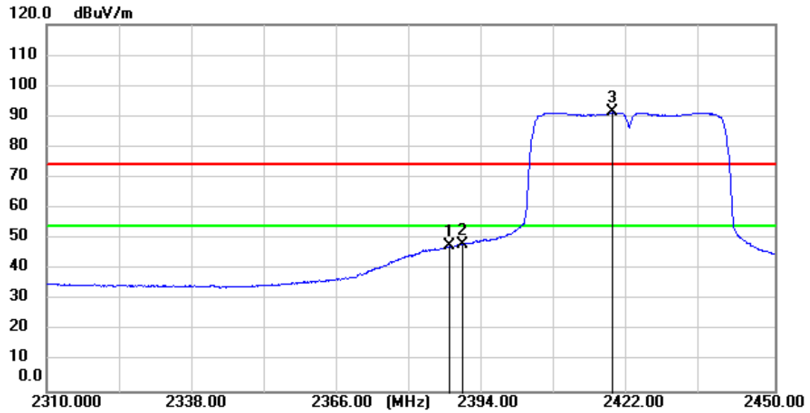
11n(HT40)_TX_CH_03_Vertical_Average
