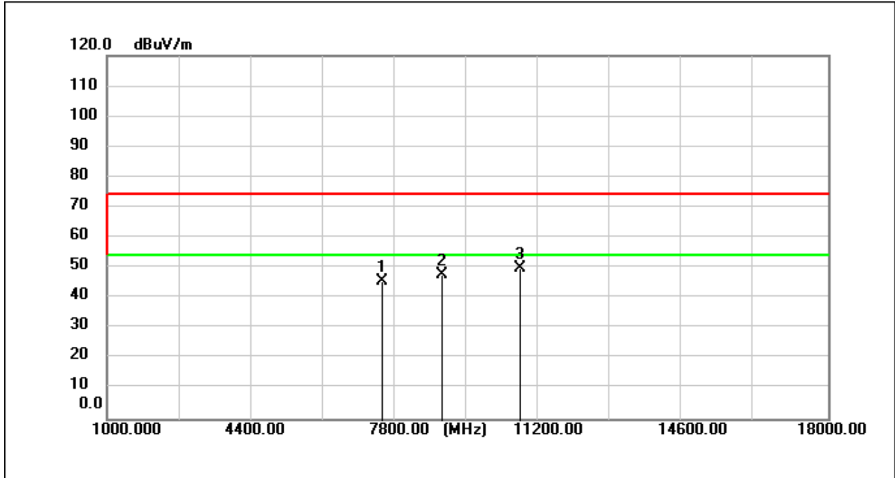
11b_TX_CH_01_Vertical
