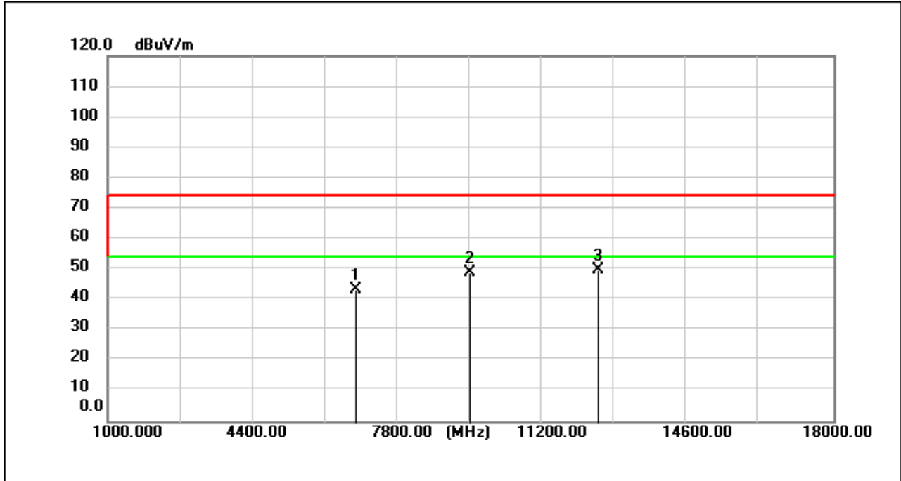
11b_TX_CH_11_Horizontal
