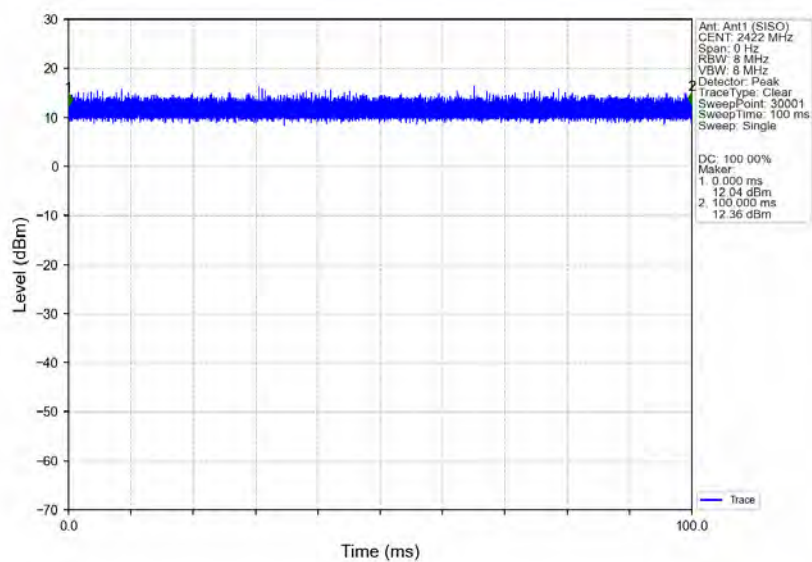
802.11n(HT40)_LCH_2422MHz_Ant1 (SISO)_NTNV
