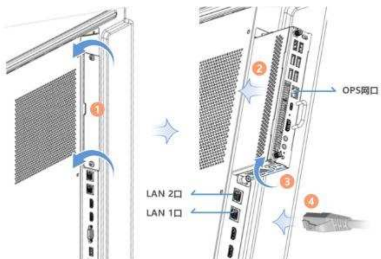
OPS 安装示意图
