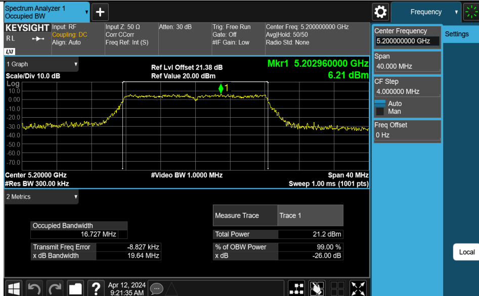
11A-Ant1-5200
