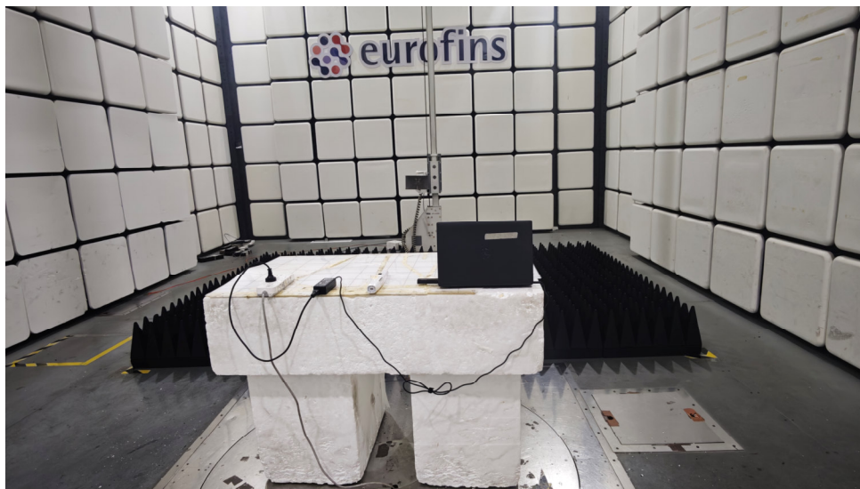
1GHz-18GHz
