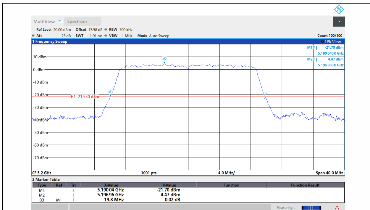
11AC20MIMO-Ant1-5200
