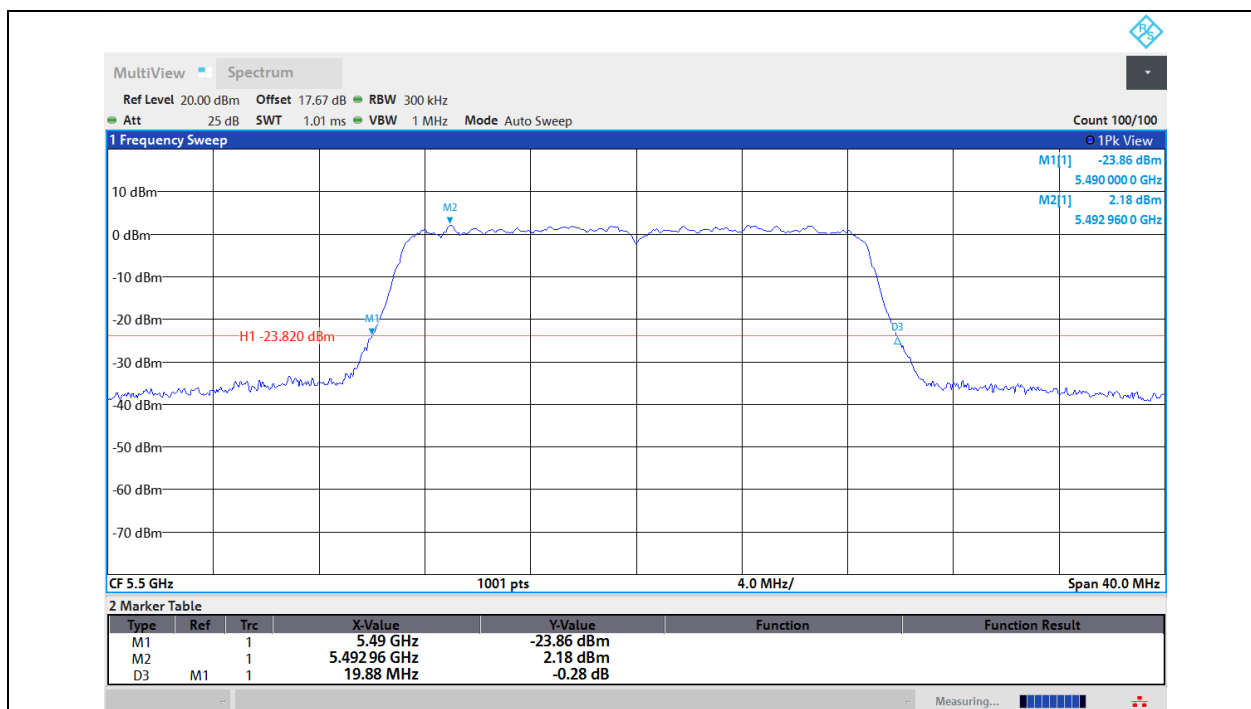
11N20MIMO-Ant1-5500
