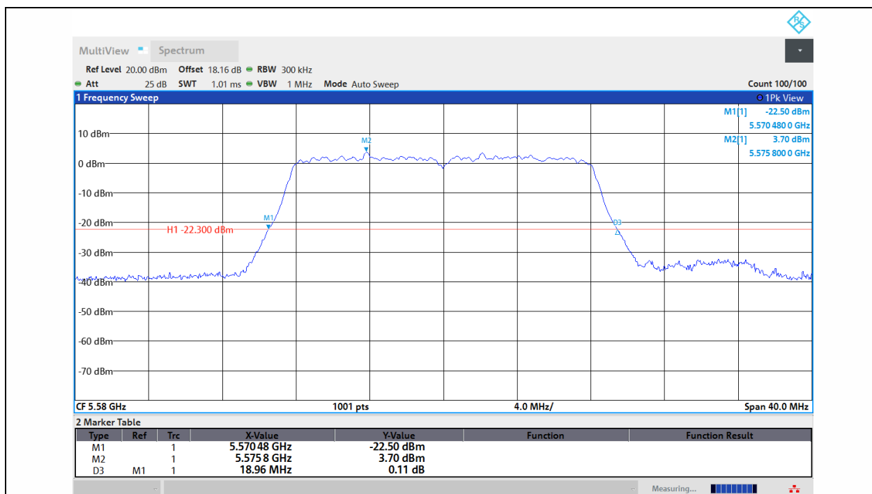
11A-Ant1-5580
