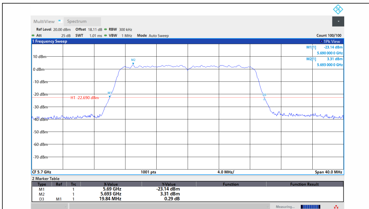
11N20MIMO-Ant1-5700
