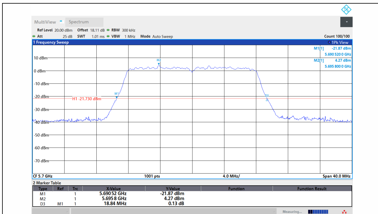
11A-Ant1-5700
