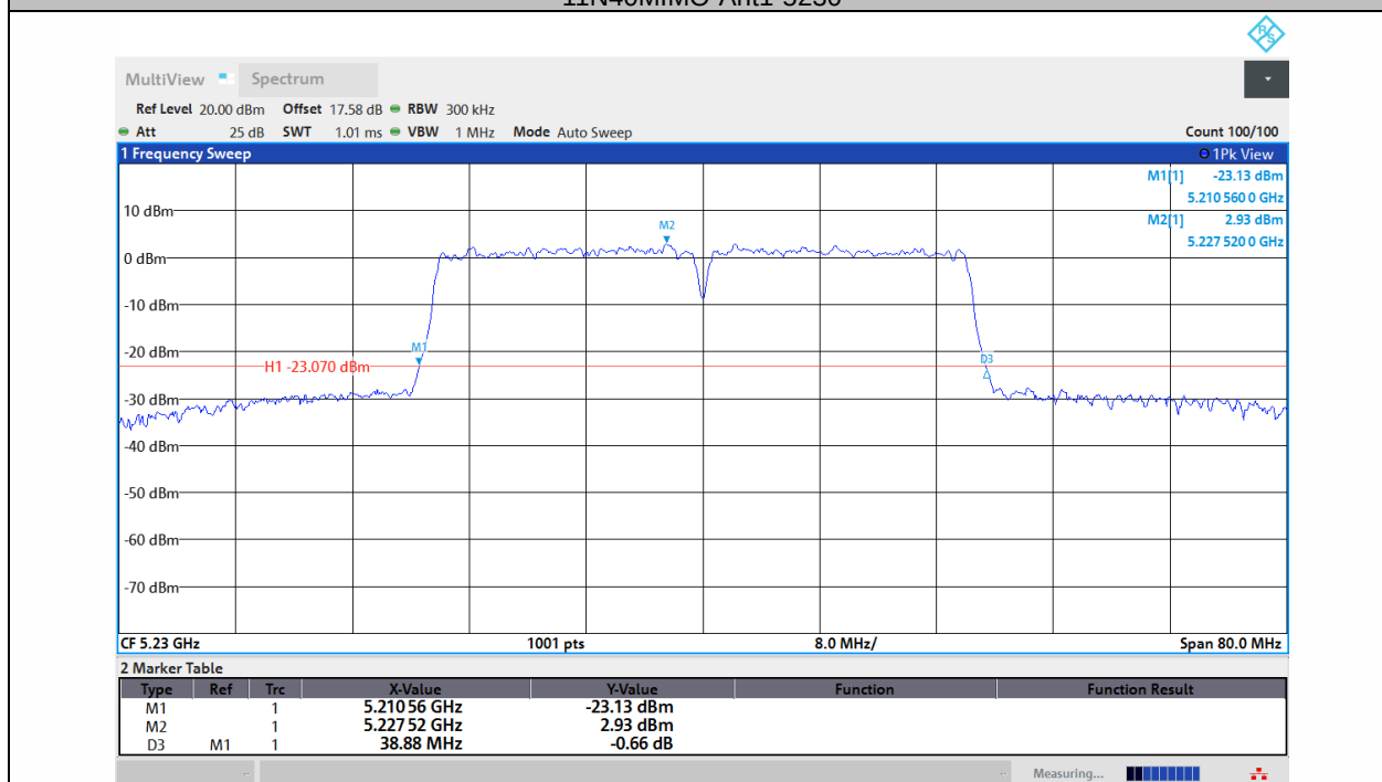
11N40MIMO-Ant2-5230
