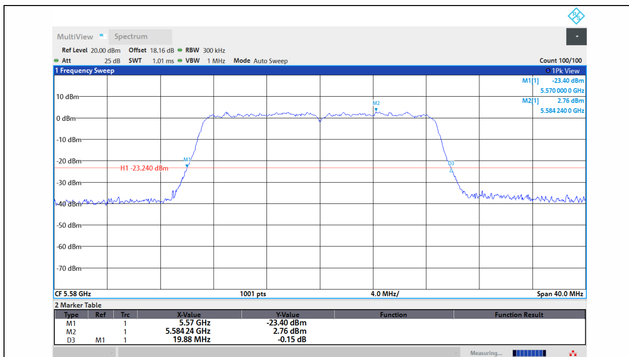
11N20MIMO-Ant1-5580
