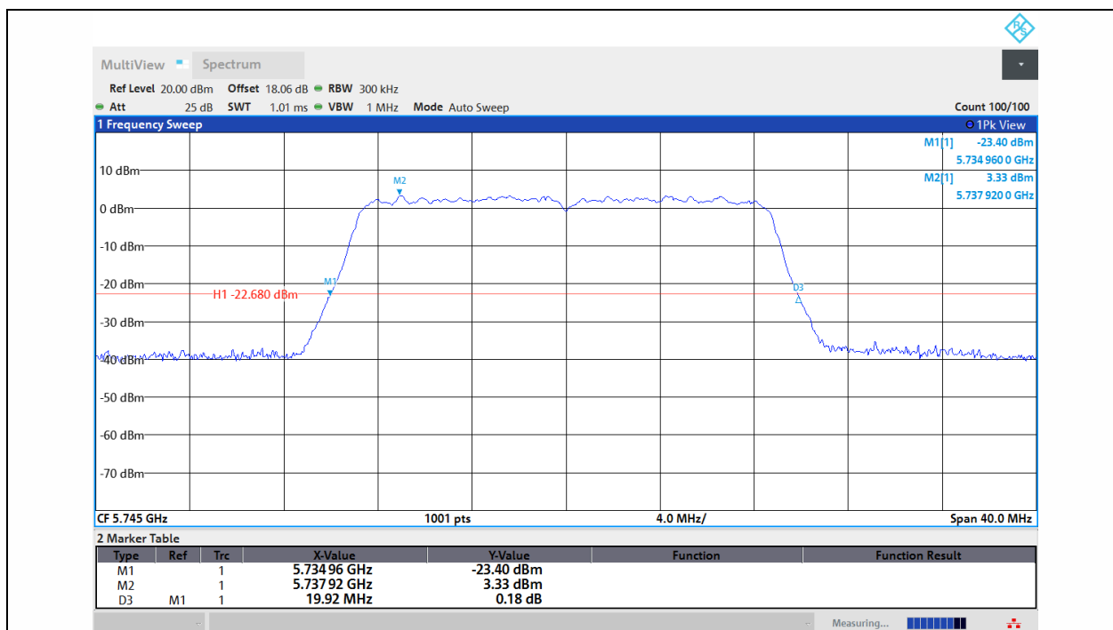
11N20MIMO-Ant1-5745
