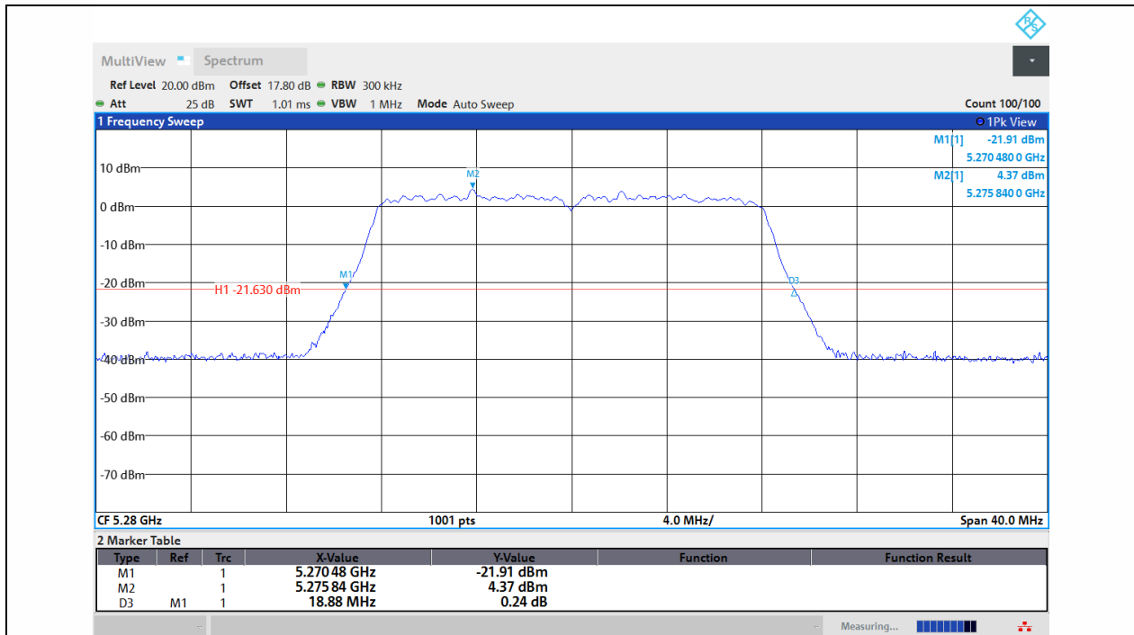
11A-Ant1-5280
