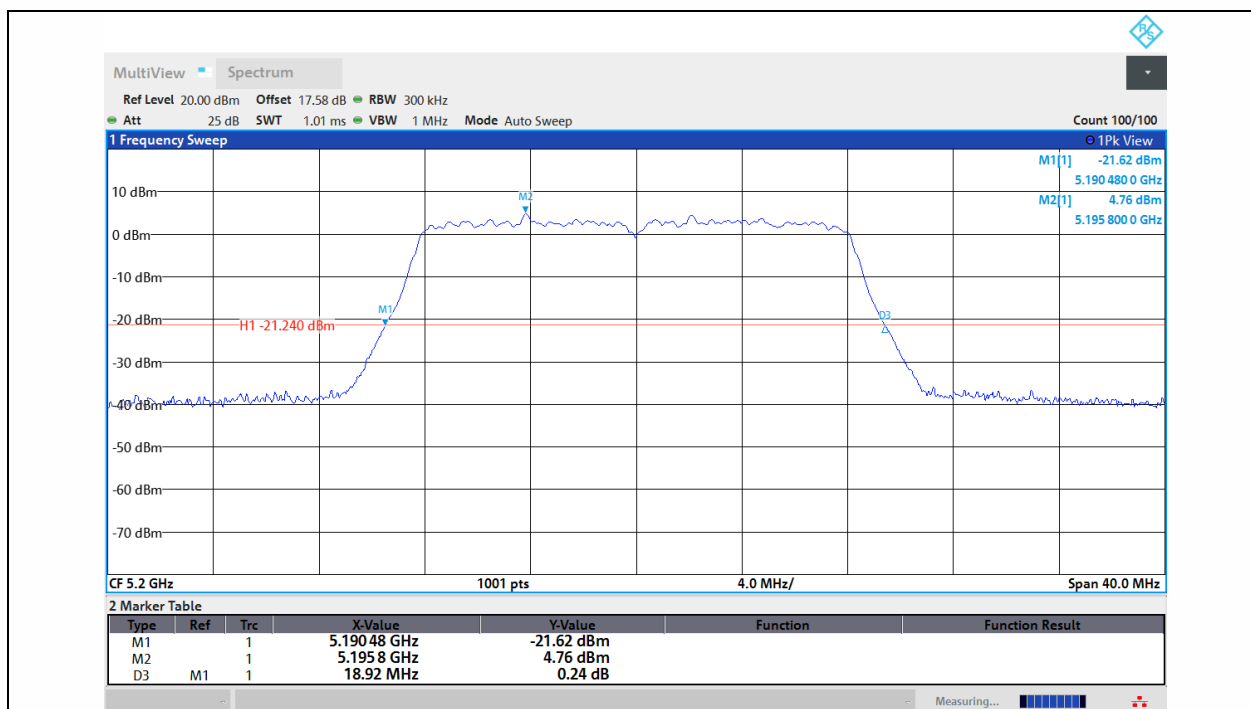
11A-Ant1-5200
