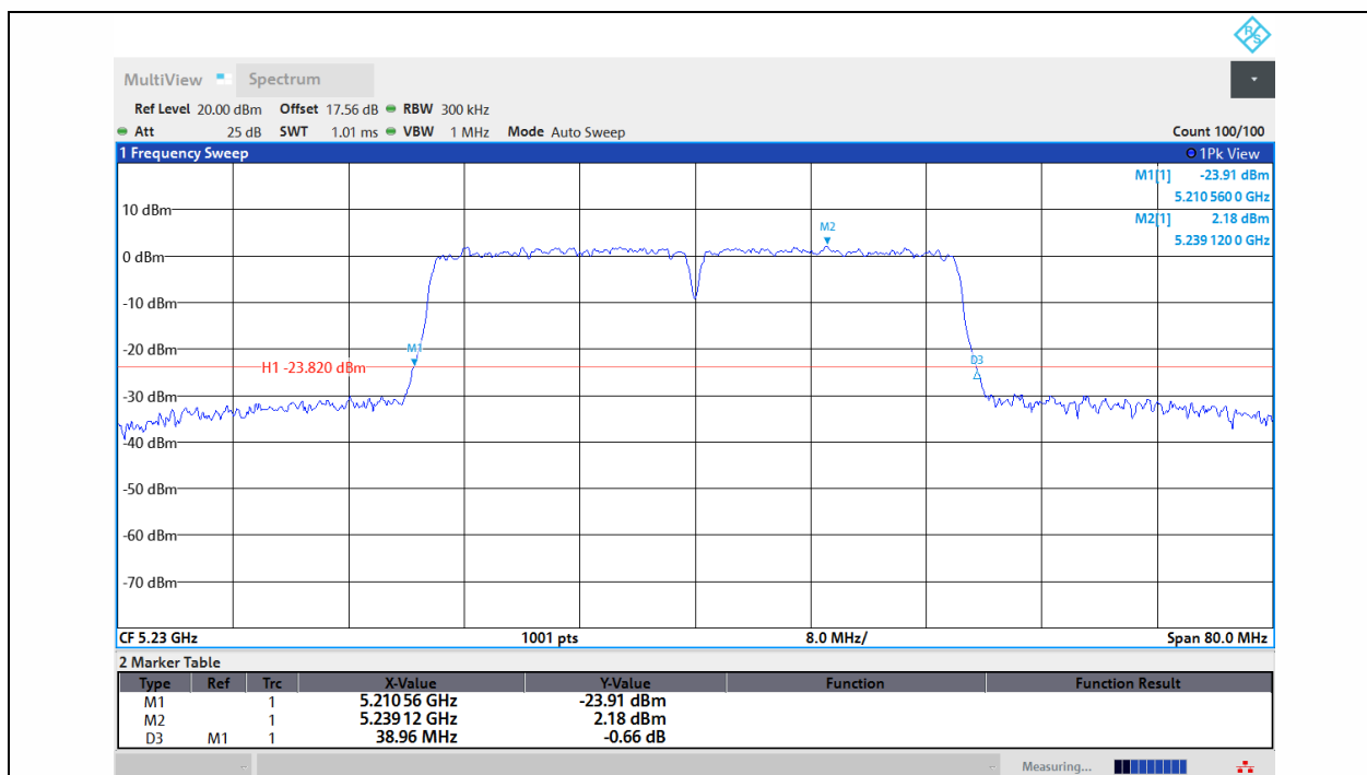
11N40MIMO-Ant1-5230
