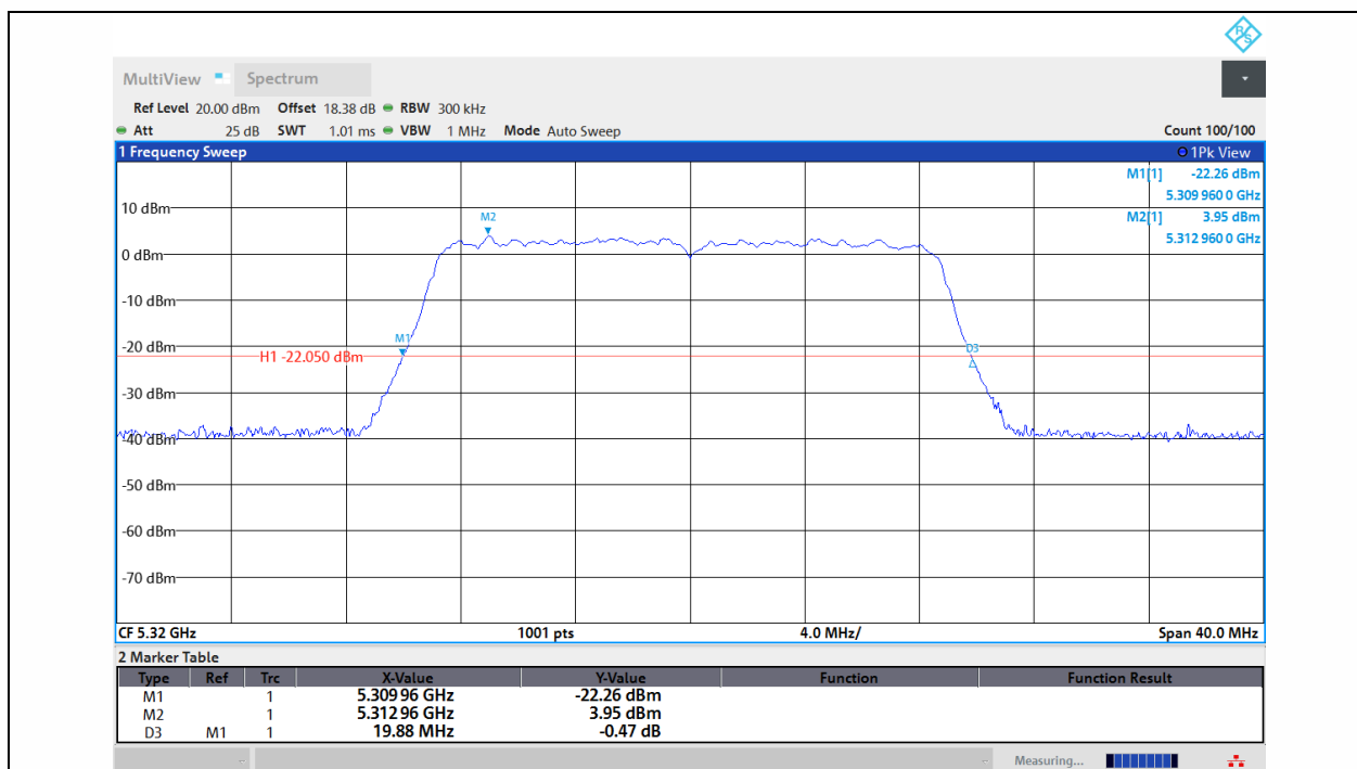
11N20MIMO-Ant1-5320
