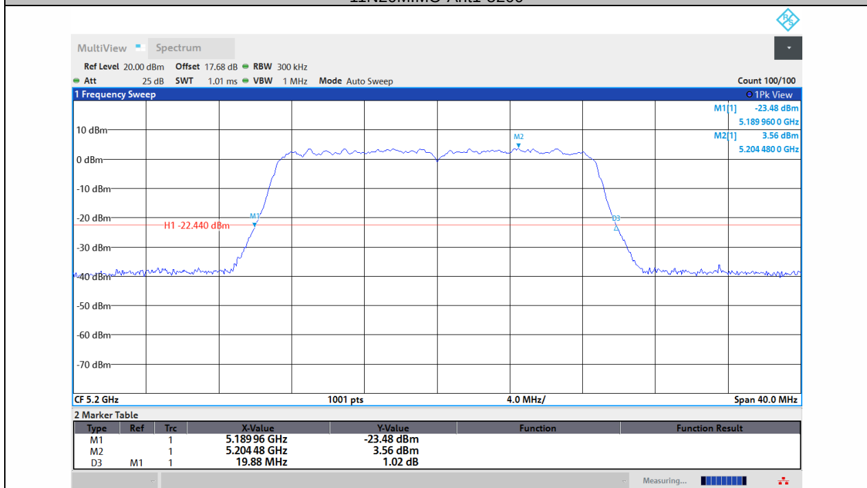
11N20MIMO-Ant2-5200
