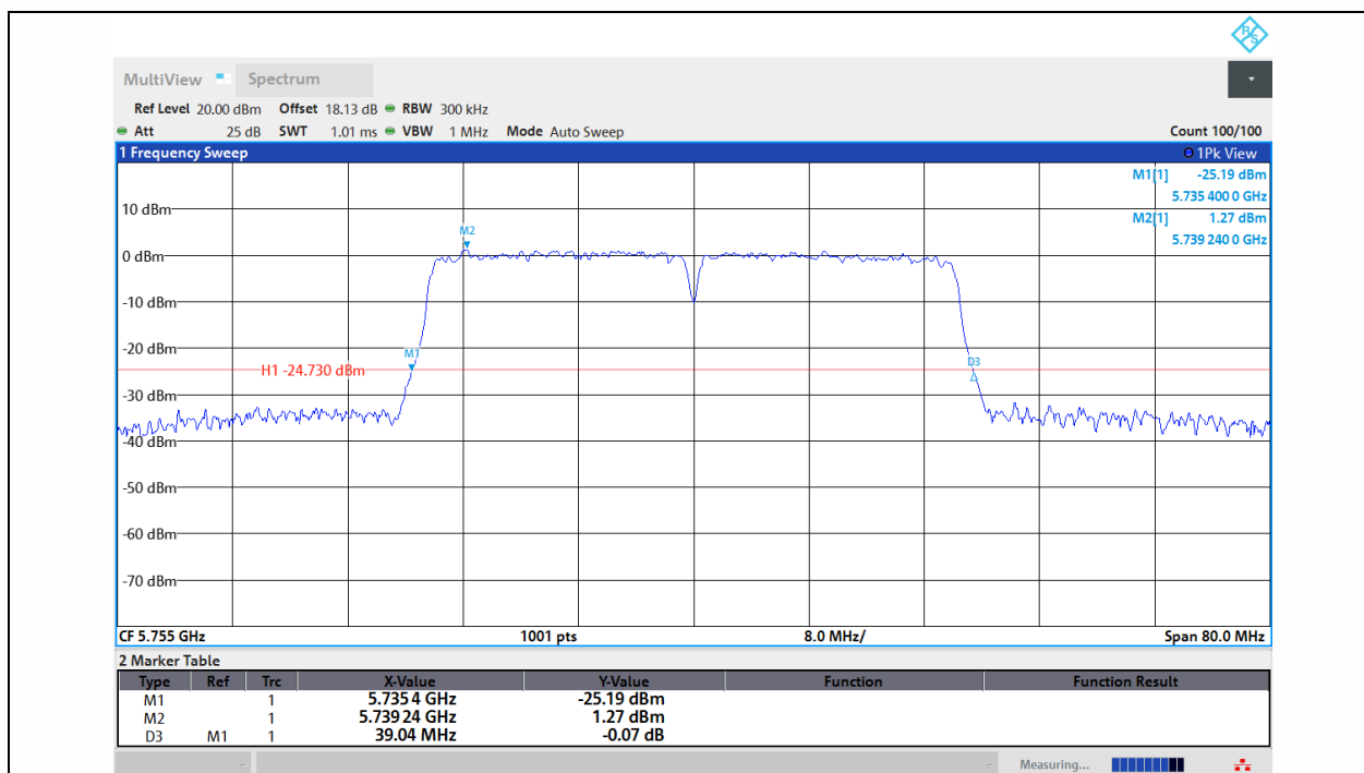
11N40MIMO-Ant1-5755
