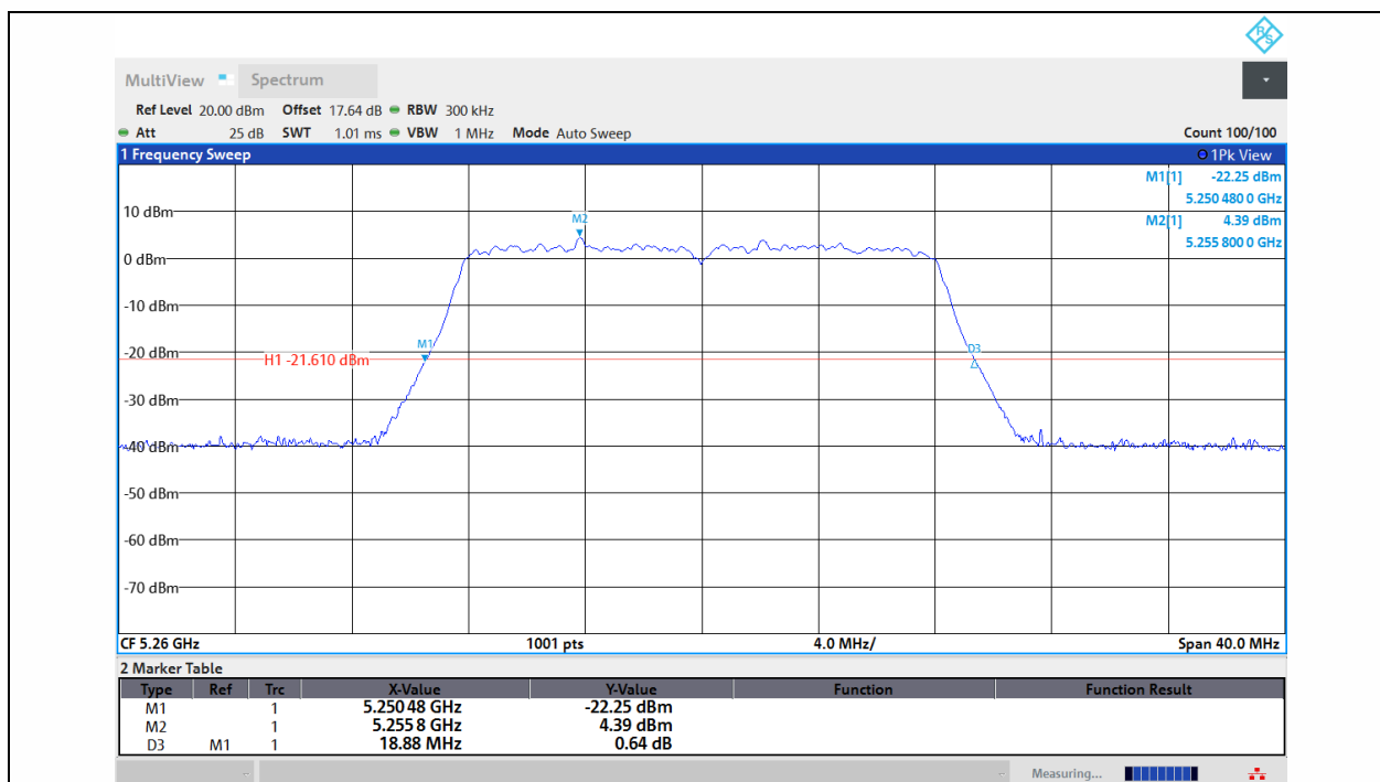
11A-Ant1-5260
