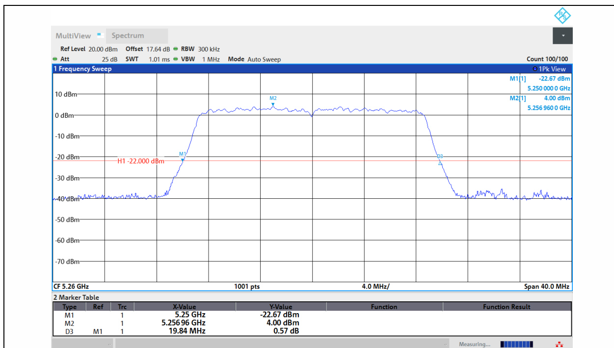
11AC20MIMO-Ant1-5260
