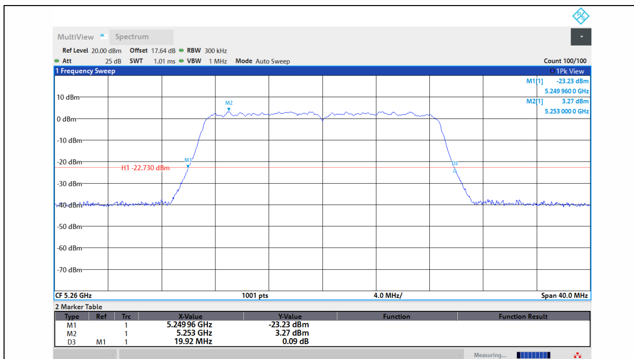
11N20MIMO-Ant1-5260
