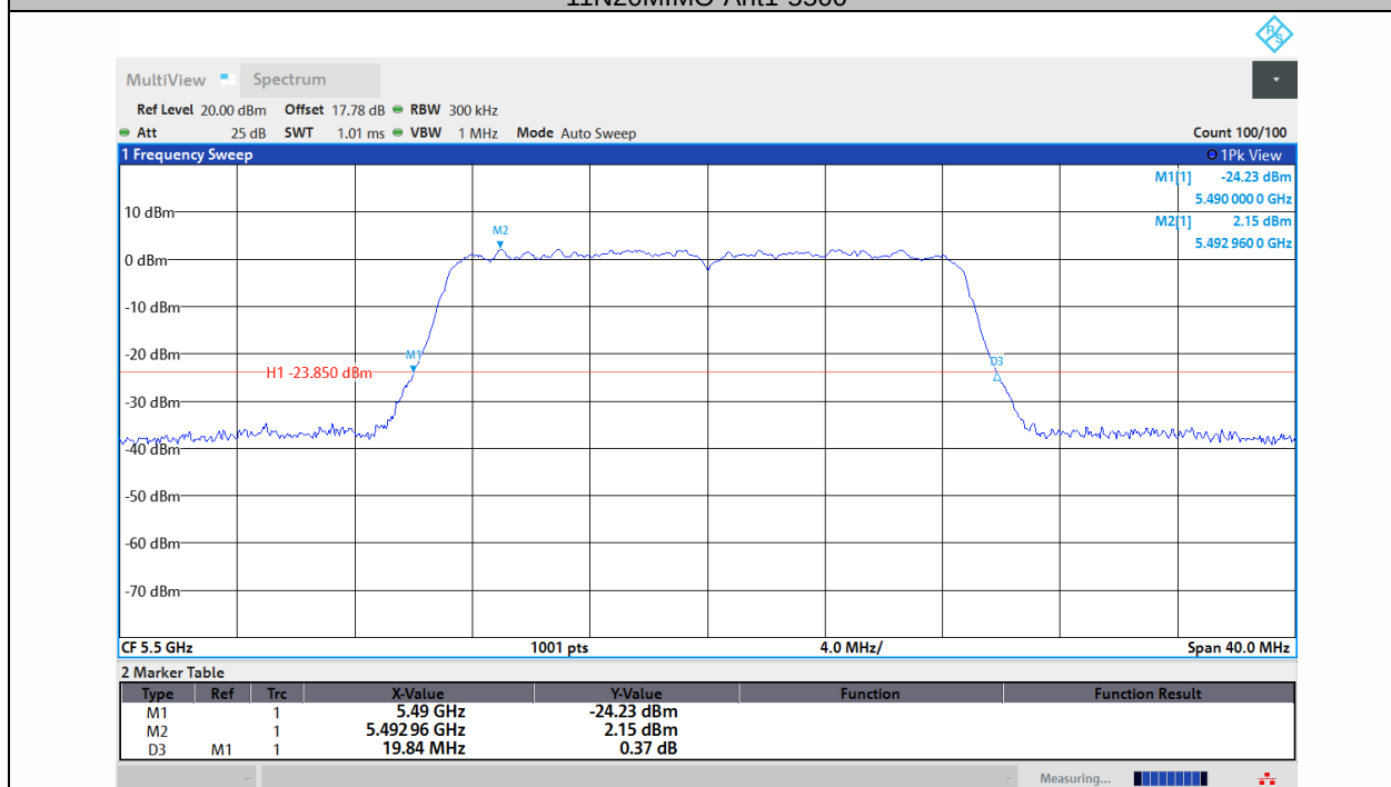
11N20MIMO-Ant2-5500
