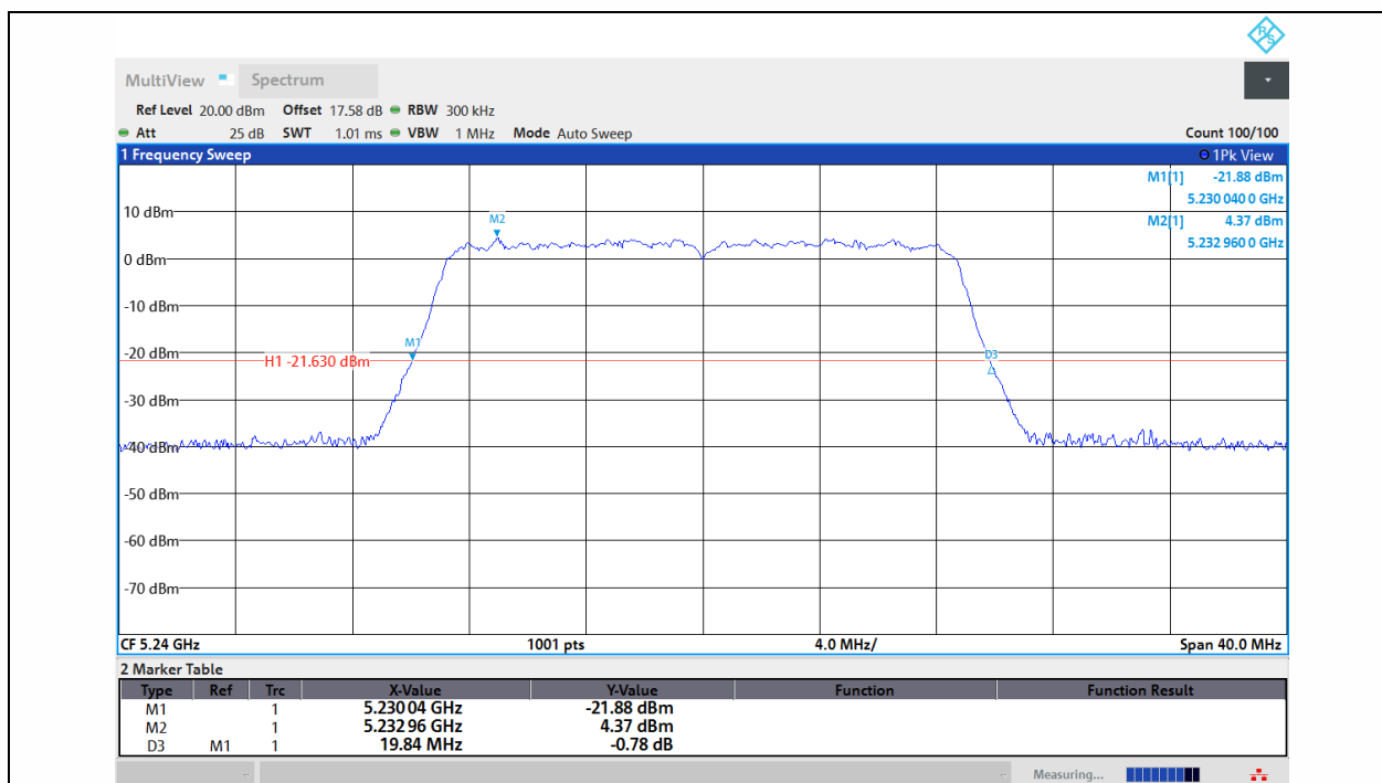
11N20MIMO-Ant1-5240
