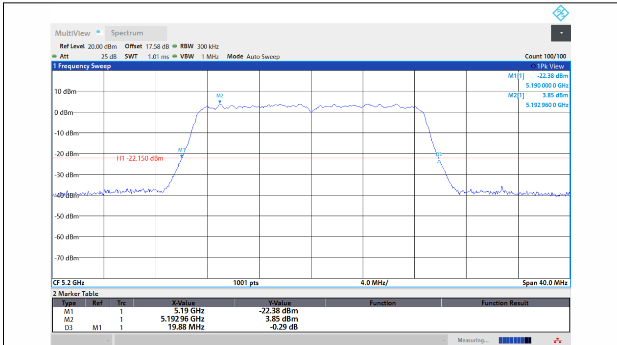
11N20MIMO-Ant1-5200
