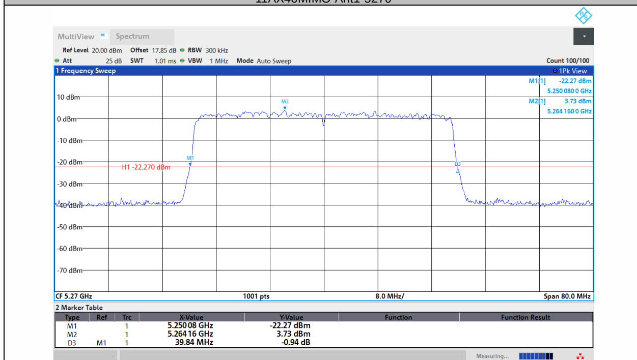
11AX40MIMO-Ant2-5270
