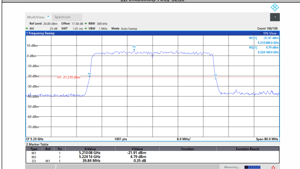
11AX40MIMO-Ant2-5230
