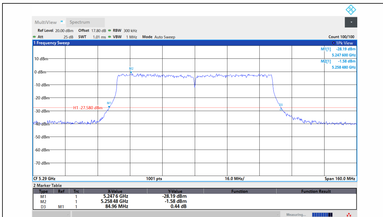
11AC80MIMO-Ant1-5290
