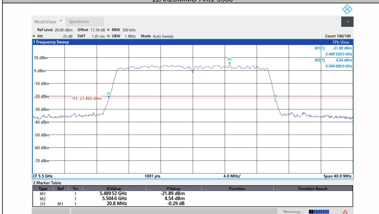
11AX20MIMO-Ant2-5500
