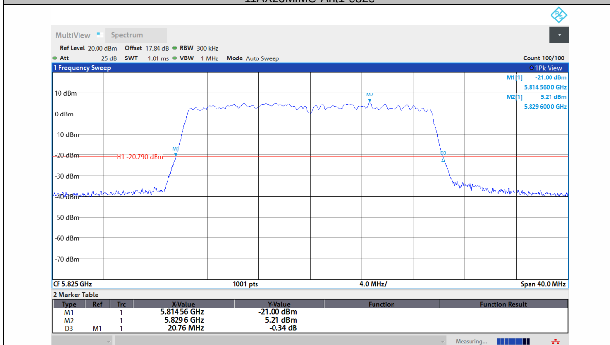
11AX20MIMO-Ant2-5825
