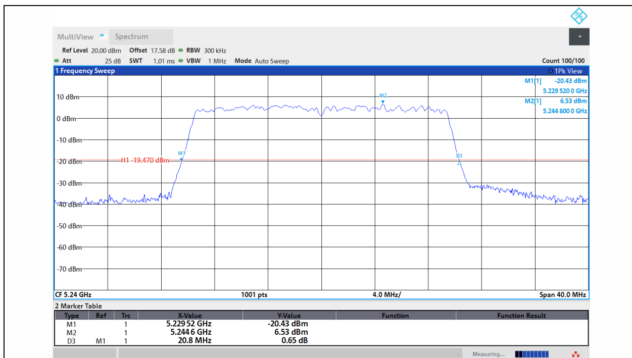
11AX20MIMO-Ant1-5240
