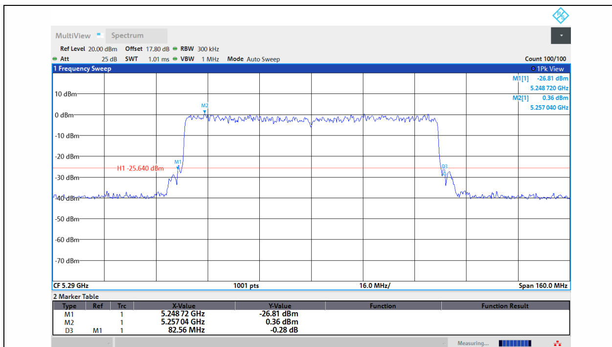
11AX80MIMO-Ant1-5290
