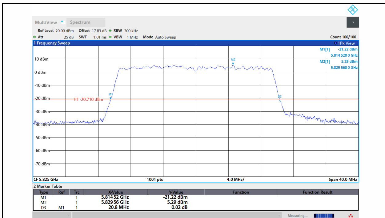
11AX20MIMO-Ant1-5825
