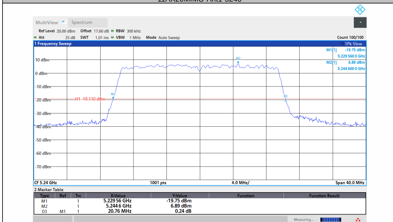
11AX20MIMO-Ant2-5240
