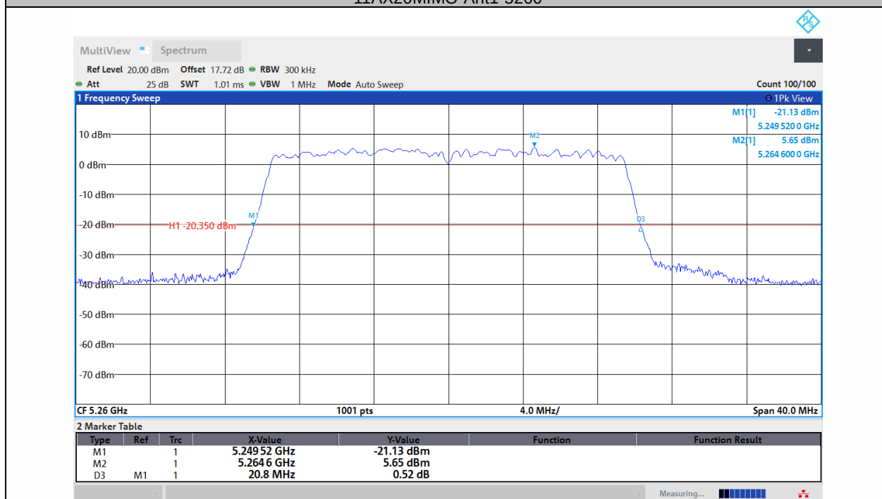
11AX20MIMO-Ant2-5260
