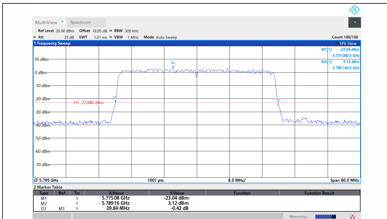
11AX40MIMO-Ant1-5795
