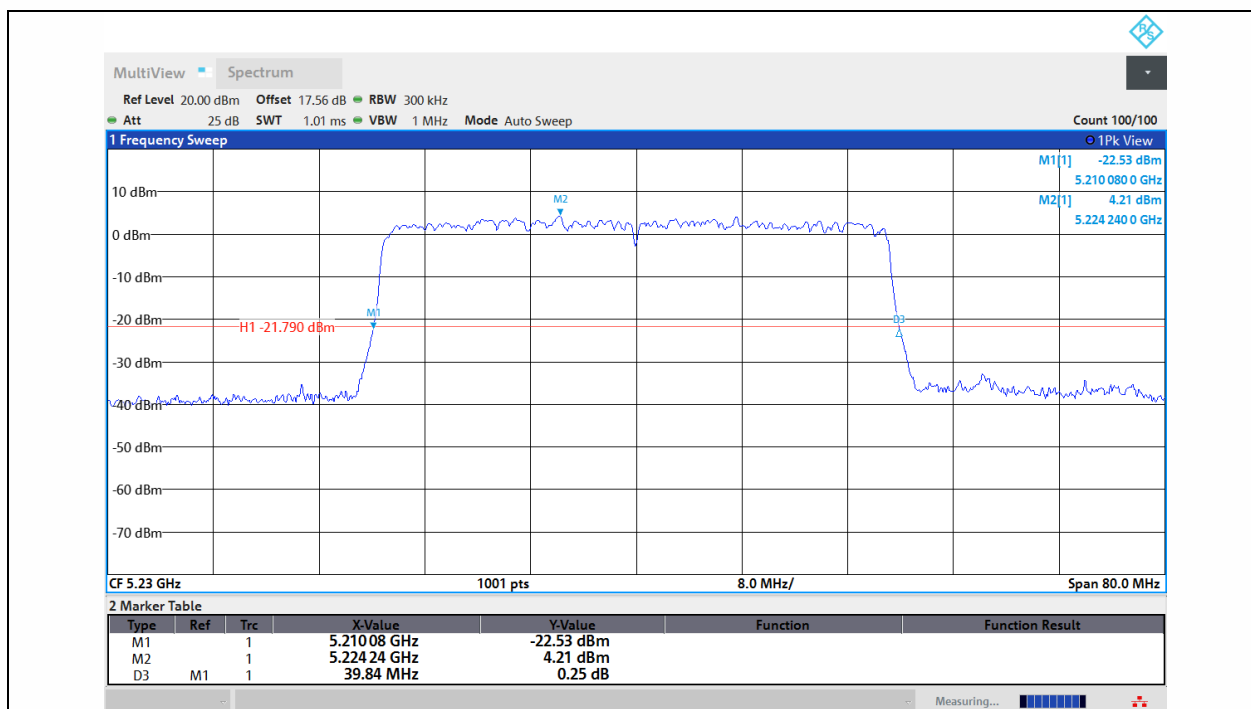
11AX40MIMO-Ant1-5230
