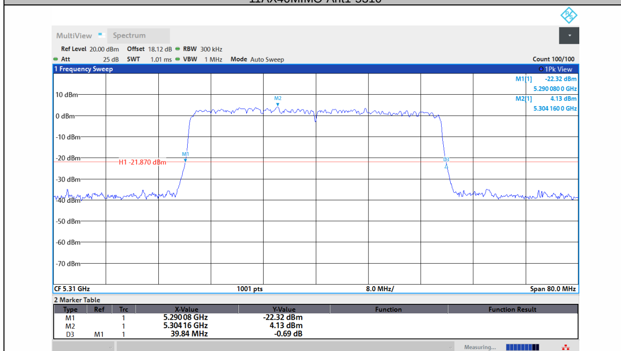
11AX40MIMO-Ant2-5310
