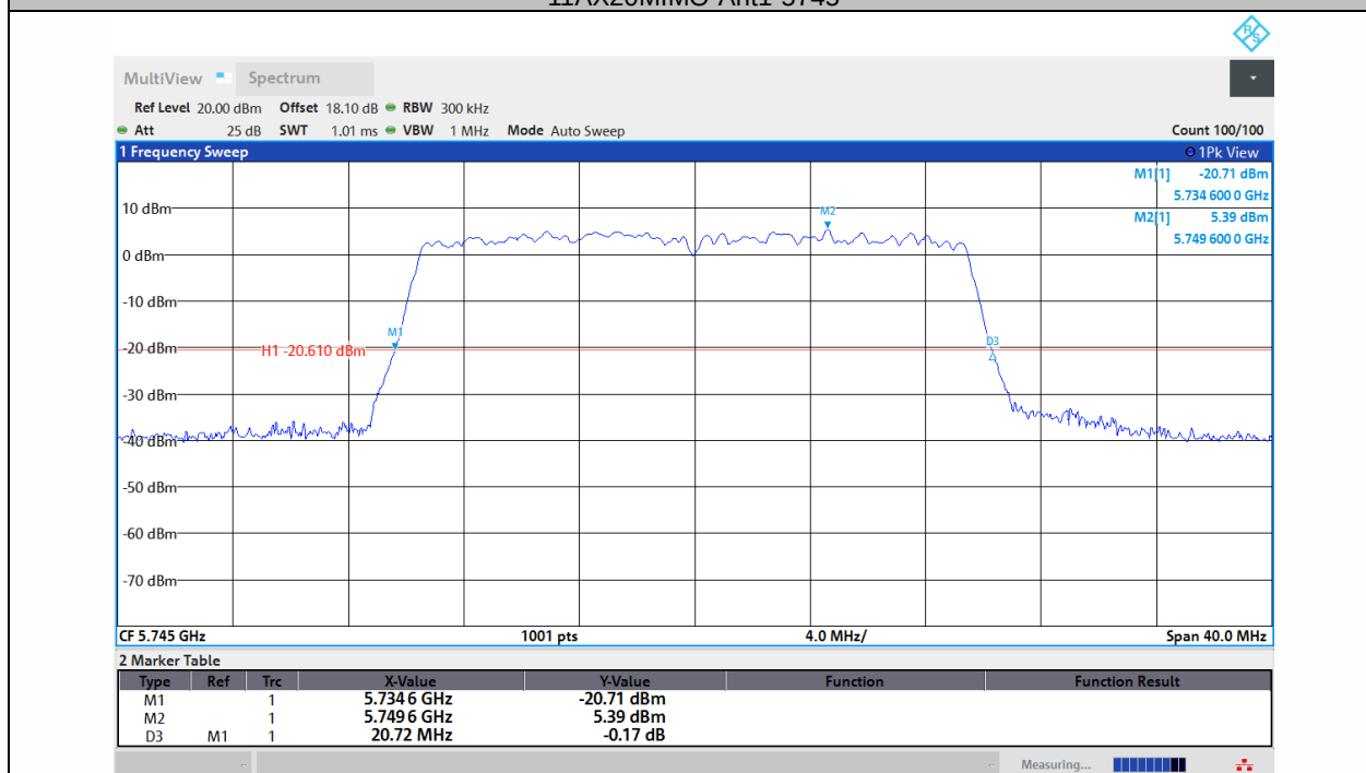
11AX20MIMO-Ant2-5745
