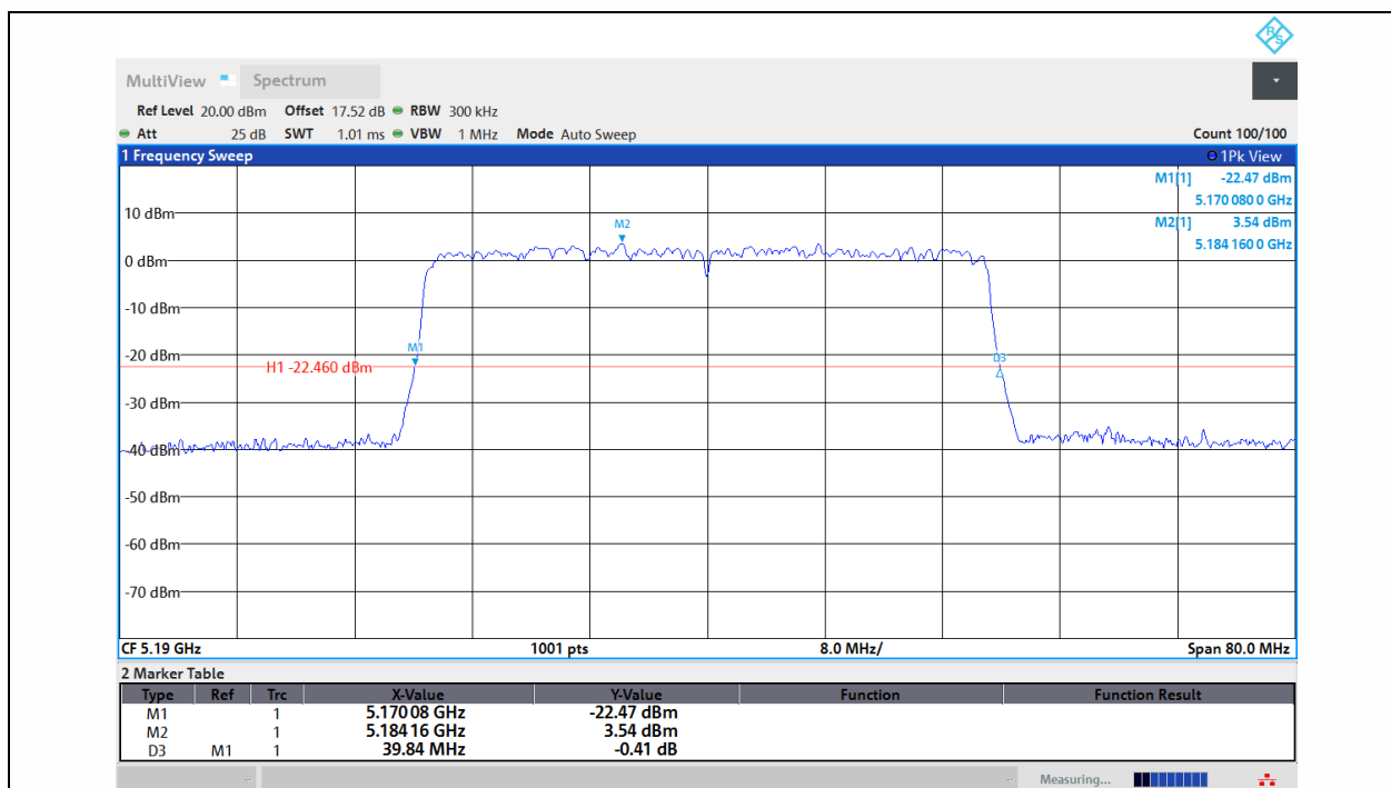
11AX40MIMO-Ant1-5190
