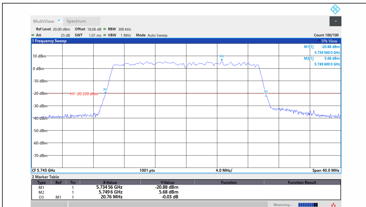
11AX20MIMO-Ant1-5745
