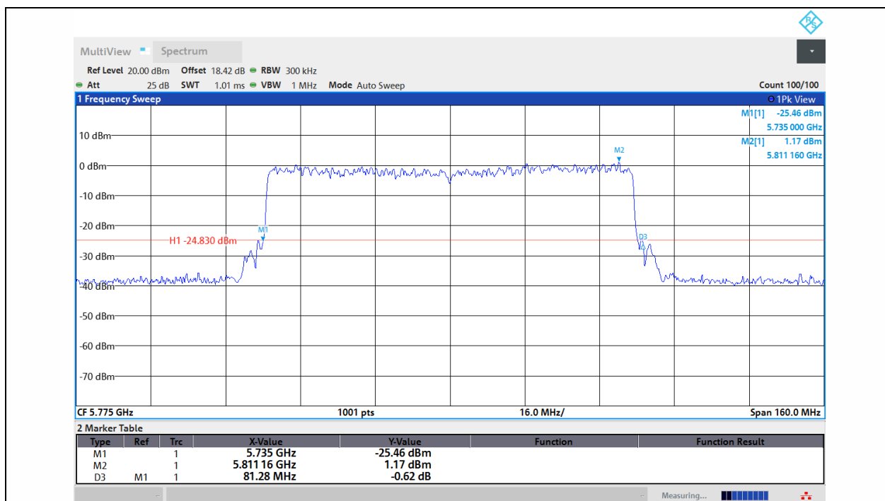
11AX80MIMO-Ant1-5775
