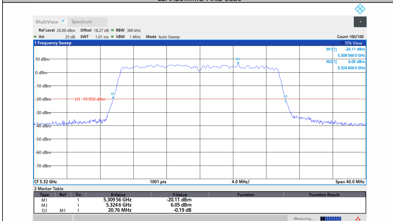
11AX20MIMO-Ant2-5320
