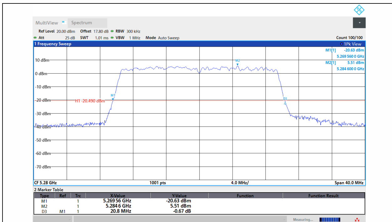
11AX20MIMO-Ant1-5280
