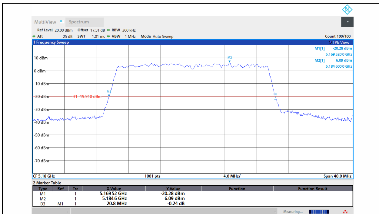
11AX20MIMO-Ant1-5180
