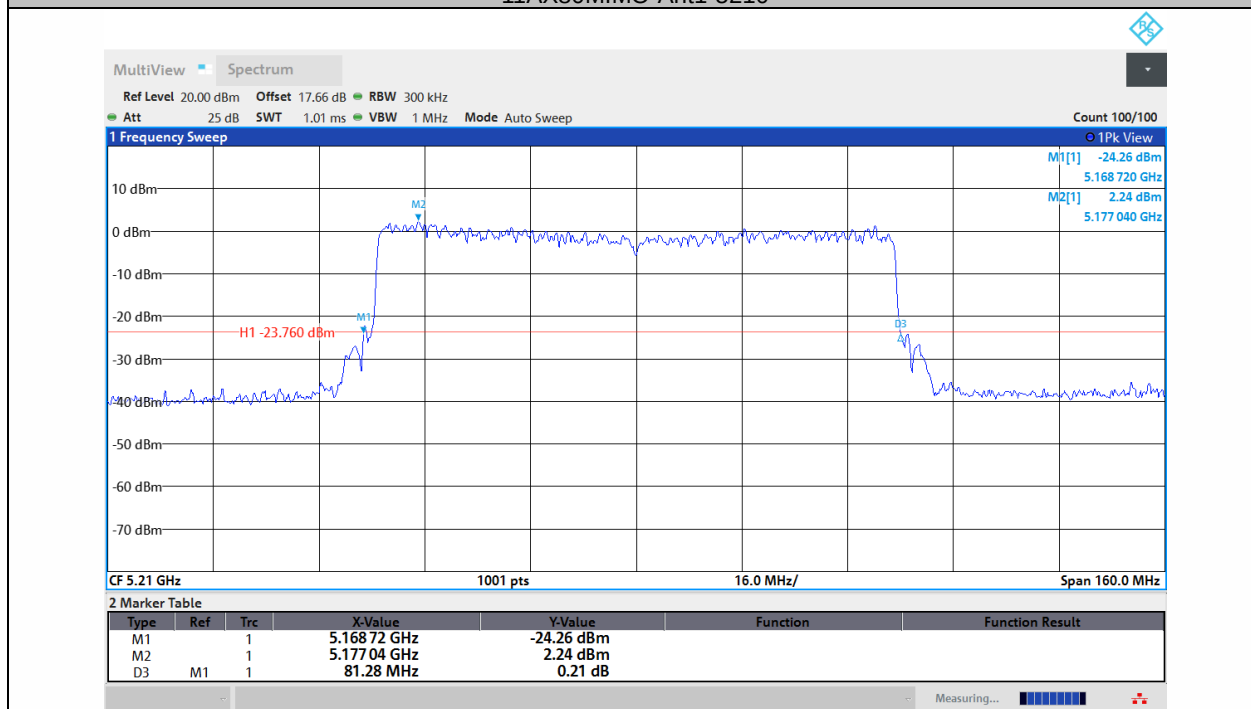
11AX80MIMO-Ant2-5210
