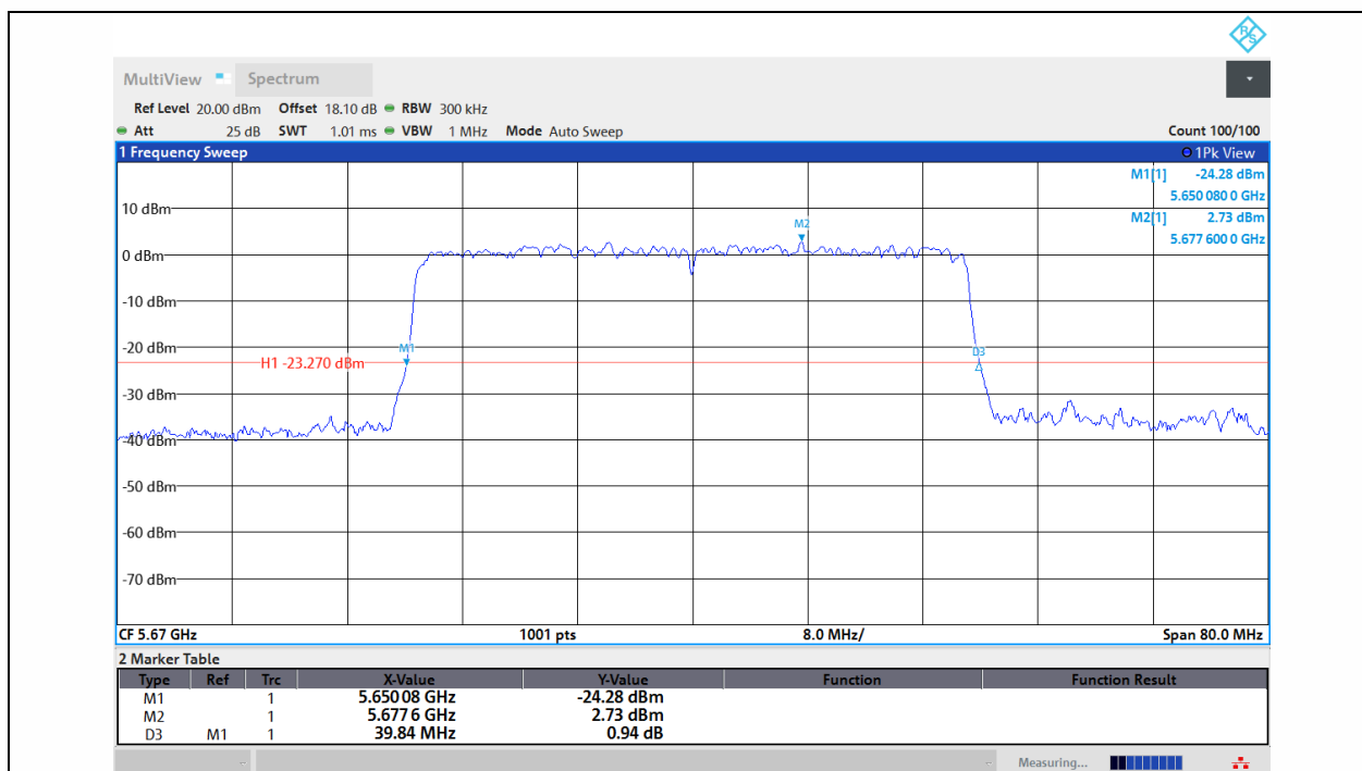
11AX40MIMO-Ant1-5670
