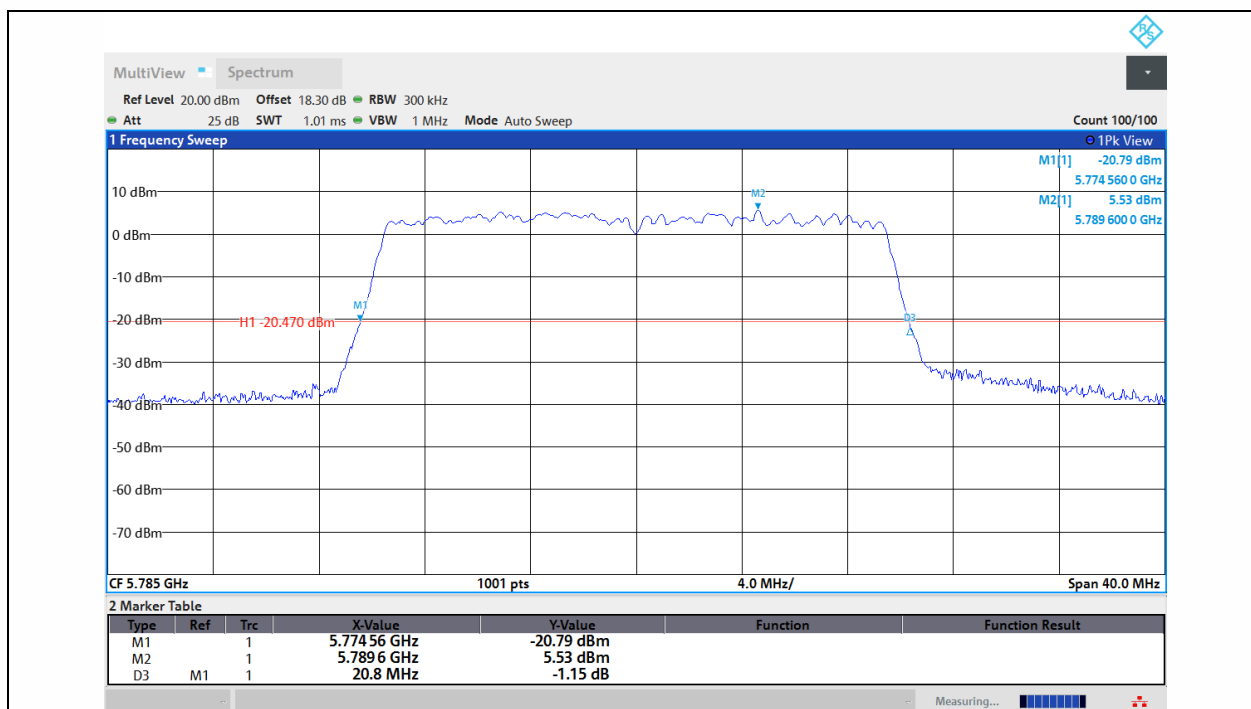
11AX20MIMO-Ant1-5785
