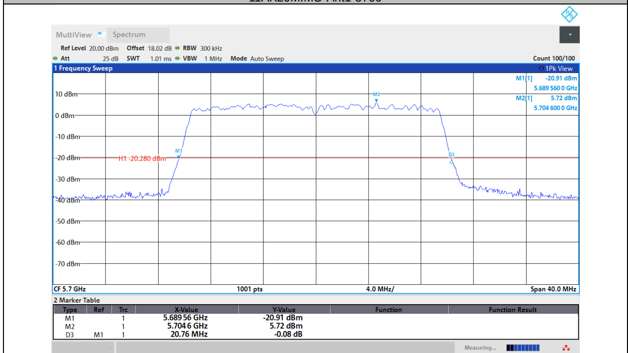
11AX20MIMO-Ant2-5700
