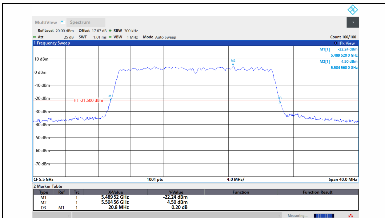
11AX20MIMO-Ant1-5500
