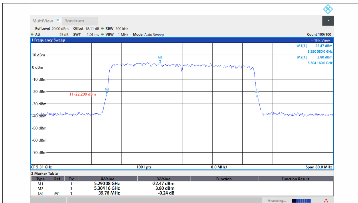
11AX40MIMO-Ant1-5310
