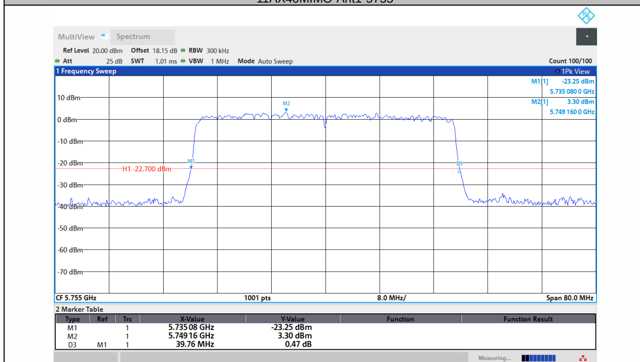
11AX40MIMO-Ant2-5755
