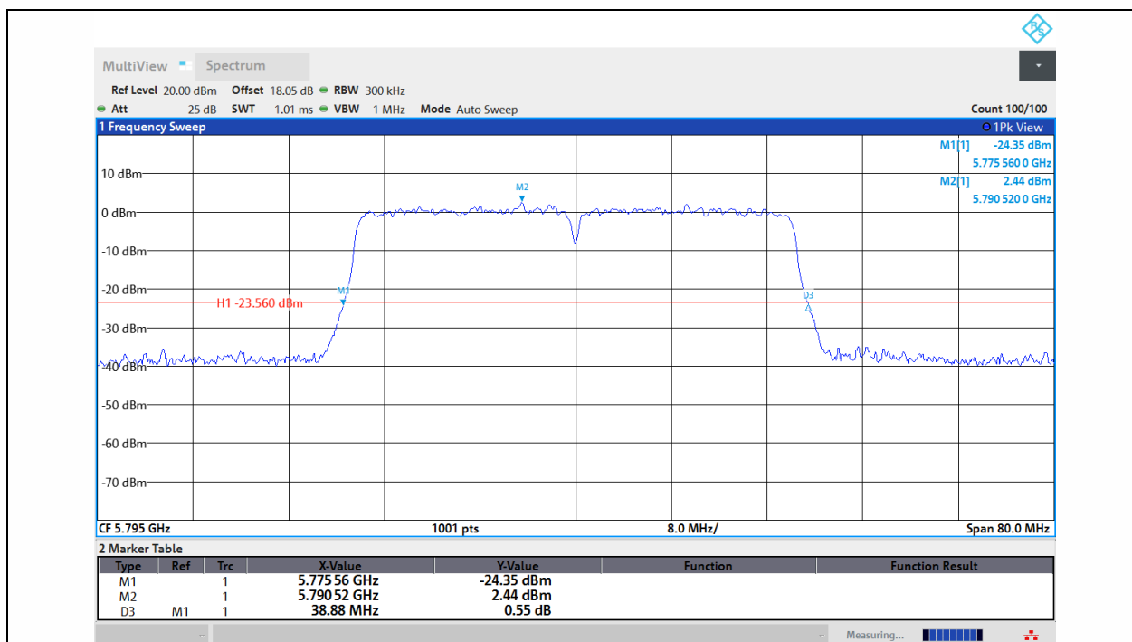
11AC40MIMO-Ant1-5795
