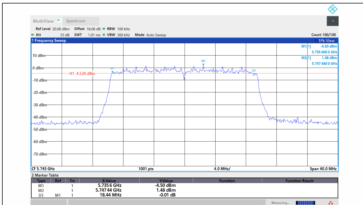
11AX20MIMO-Ant1-5745-PASS
