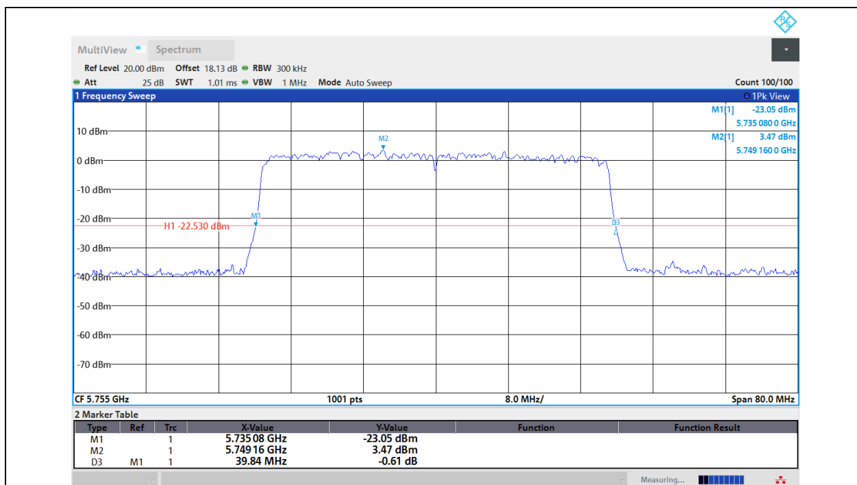
11AX40MIMO-Ant1-5755
