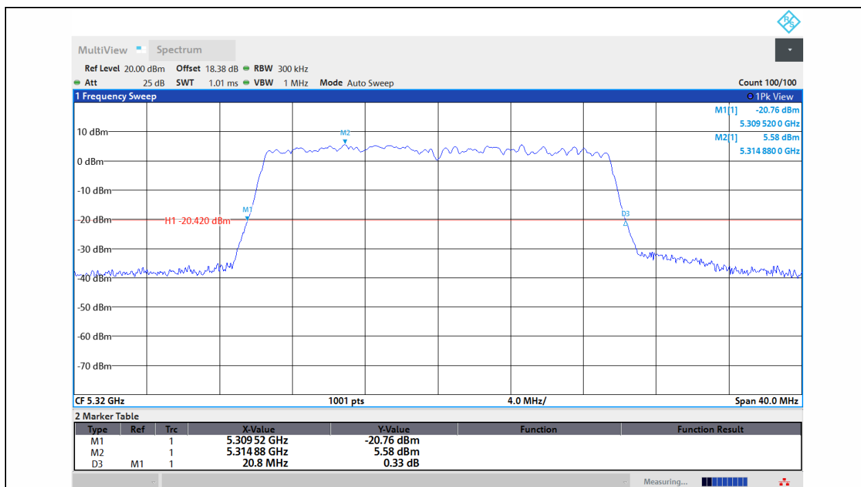
11AX20MIMO-Ant1-5320
