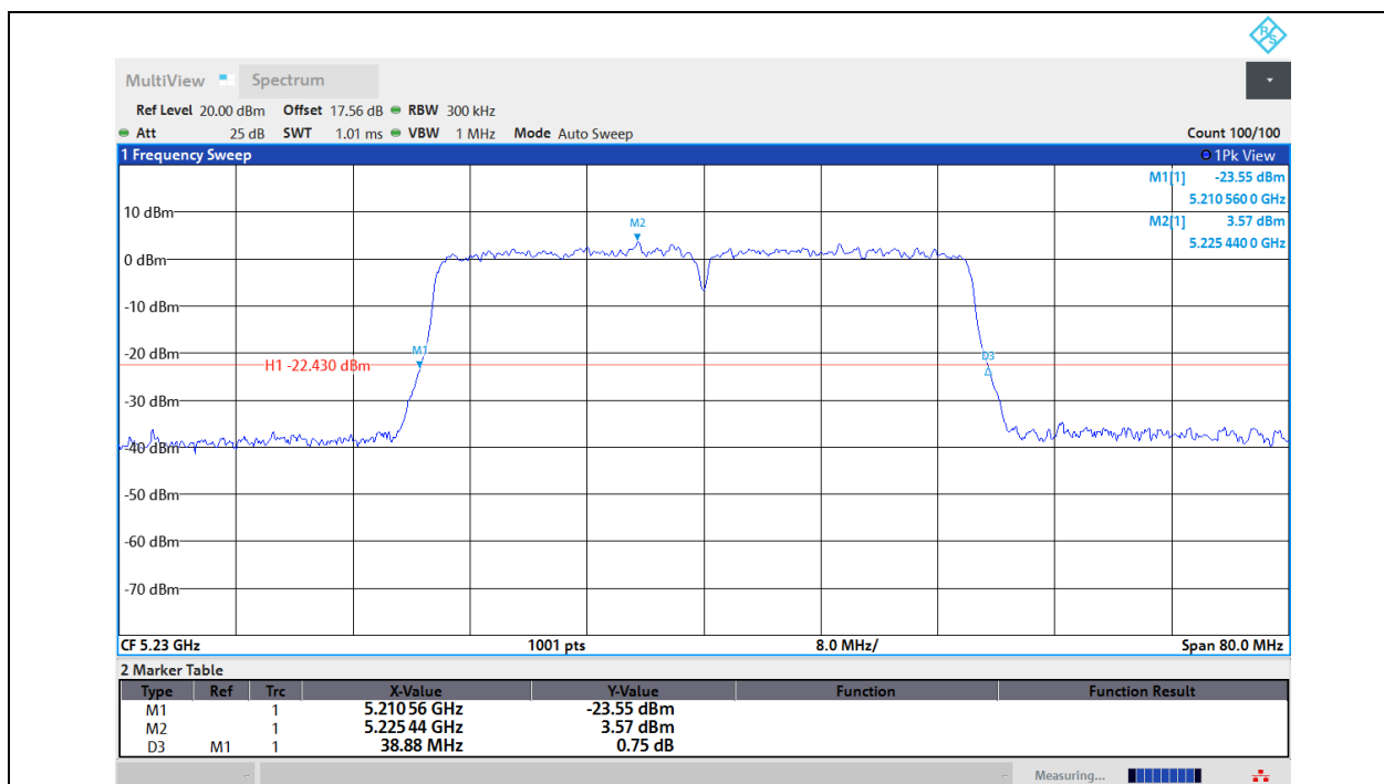
11AC40MIMO-Ant1-5230
