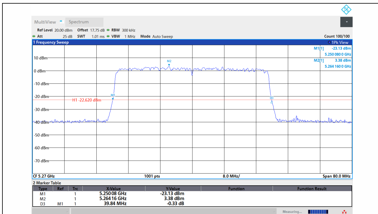
11AX40MIMO-Ant1-5270
