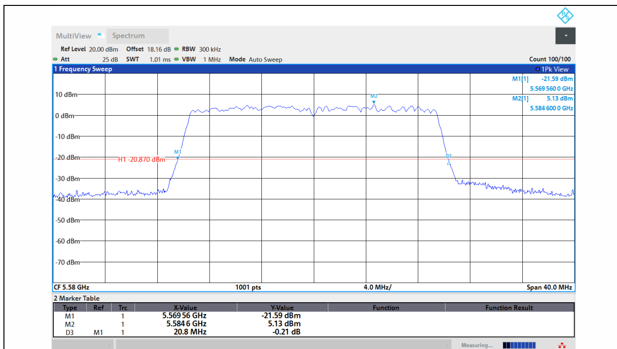
11AX20MIMO-Ant1-5580
