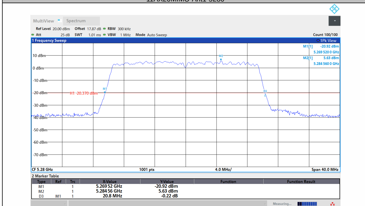
11AX20MIMO-Ant2-5280
