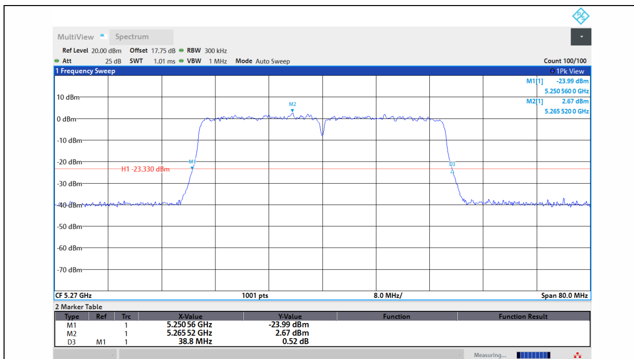
11AC40MIMO-Ant1-5270
