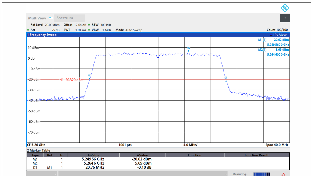
11AX20MIMO-Ant1-5260
