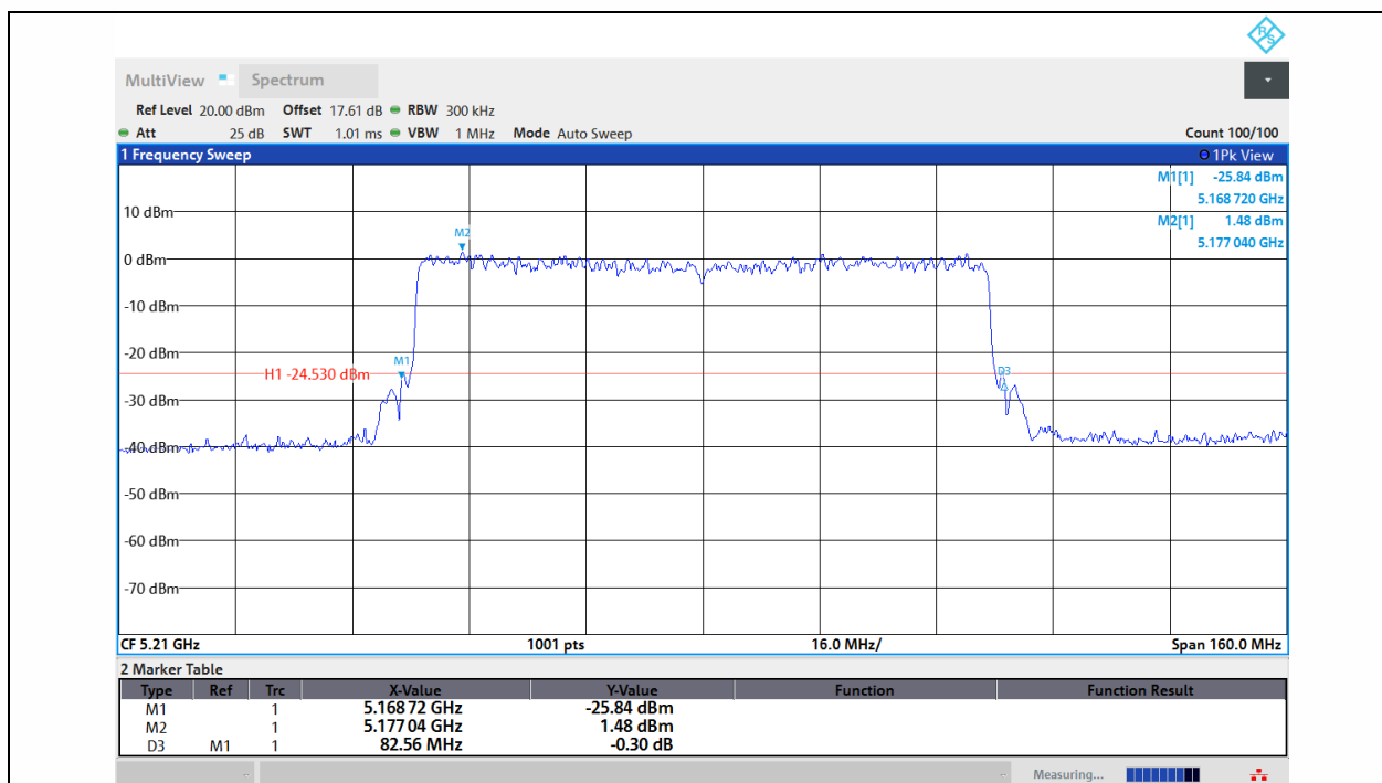
11AX80MIMO-Ant1-5210
