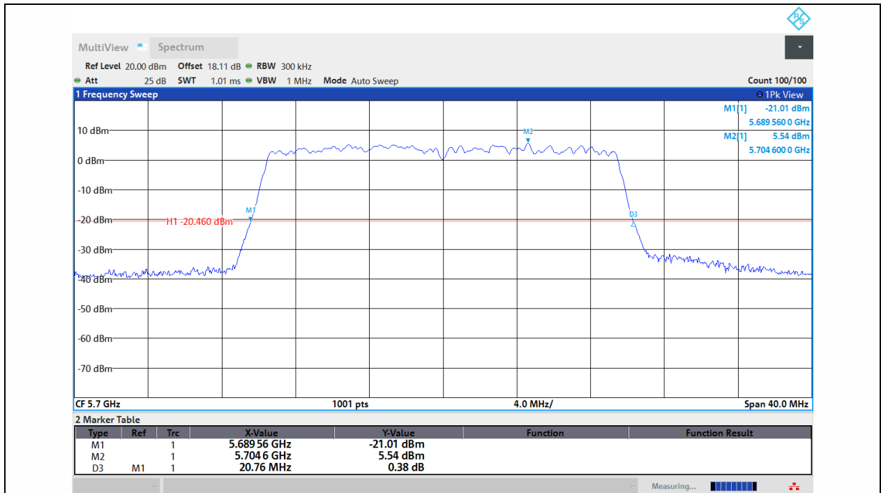
11AX20MIMO-Ant1-5700
