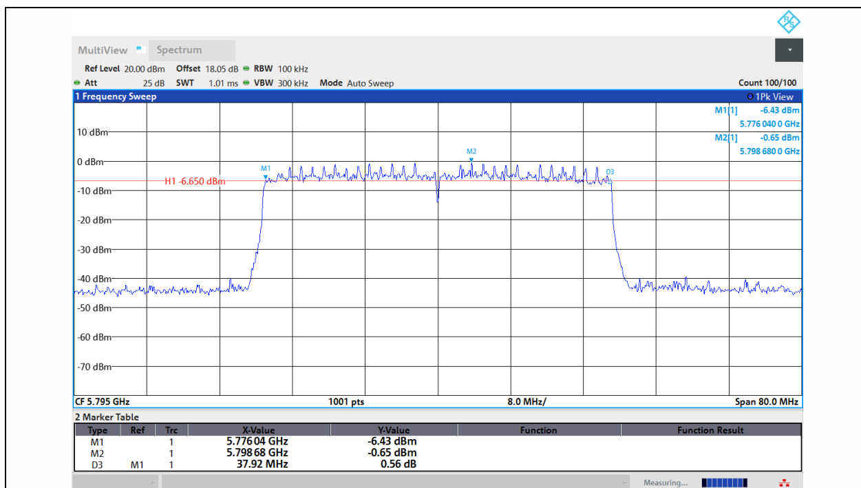
11AX40MIMO-Ant1-5795-PASS
