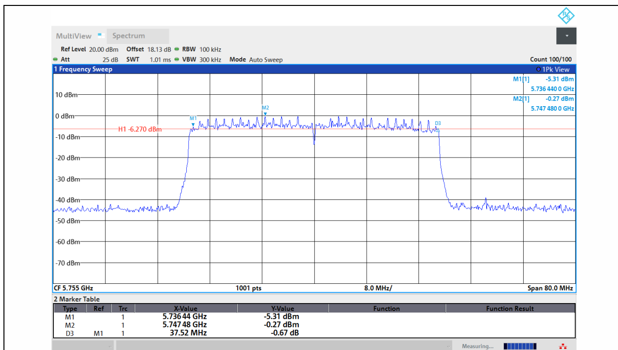
11AX40MIMO-Ant1-5755-PASS
