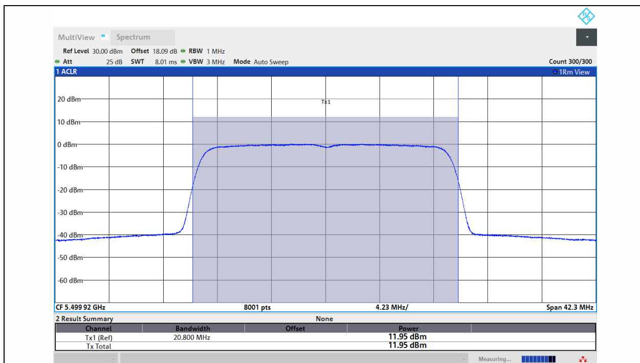
11AX20MIMO-Ant1-5500-PASS
