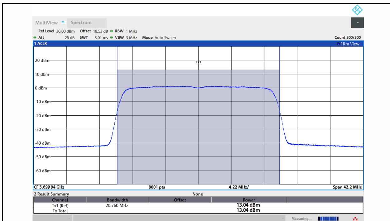
11AX20MIMO-Ant1-5700-PASS
