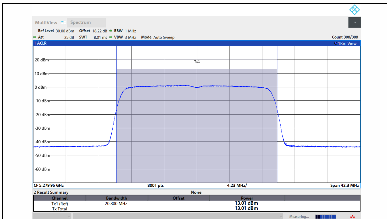
11AX20MIMO-Ant1-5280-PASS
