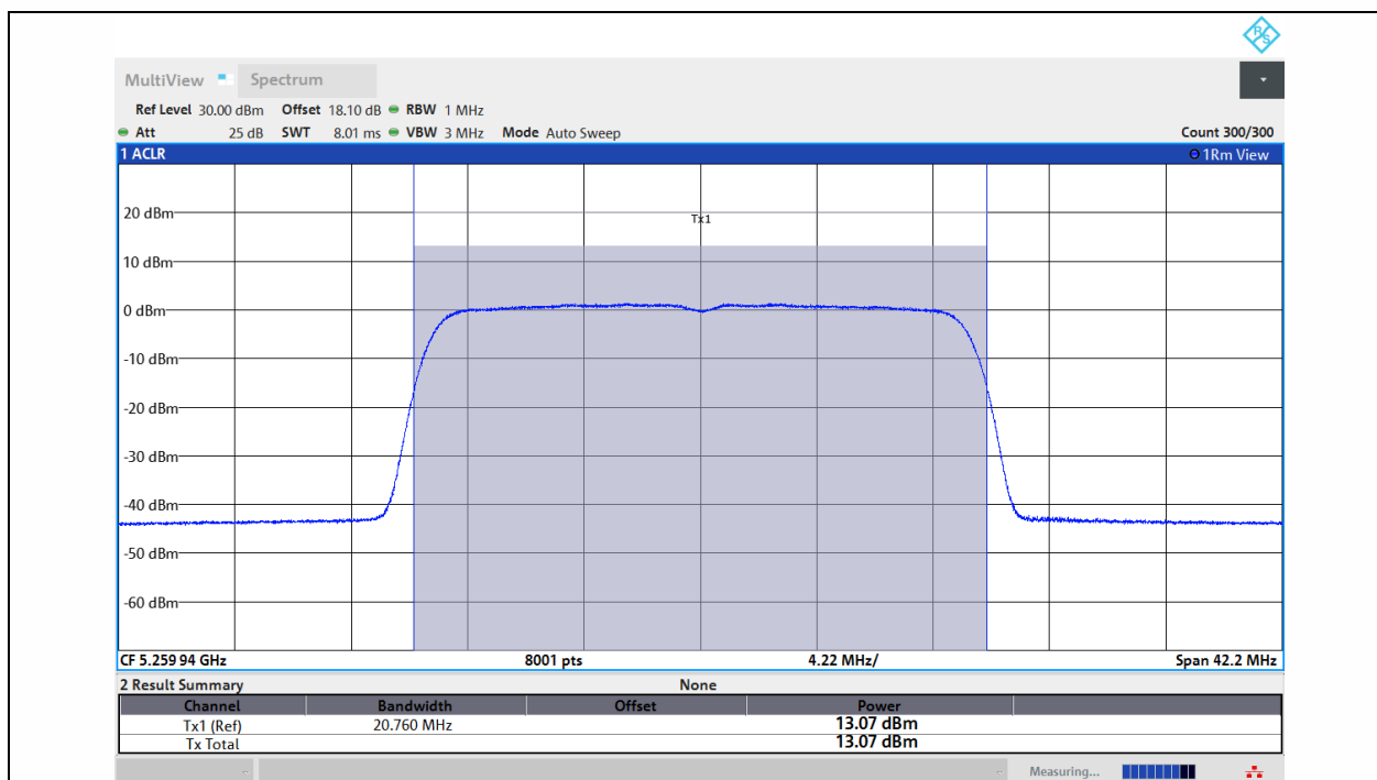
11AX20MIMO-Ant1-5260-PASS
