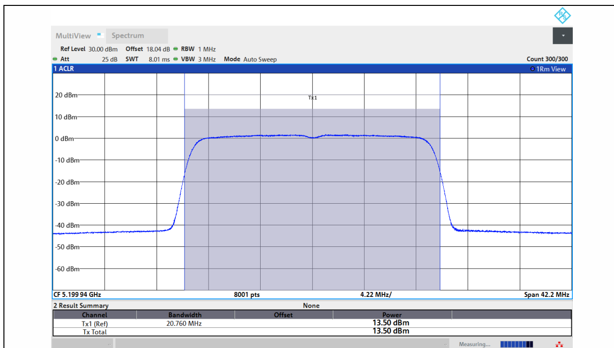
11AX20MIMO-Ant1-5200-PASS
