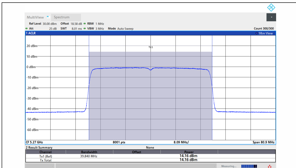
11AX40MIMO-Ant1-5270-PASS
