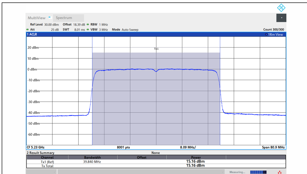
11AX40MIMO-Ant1-5230-PASS
