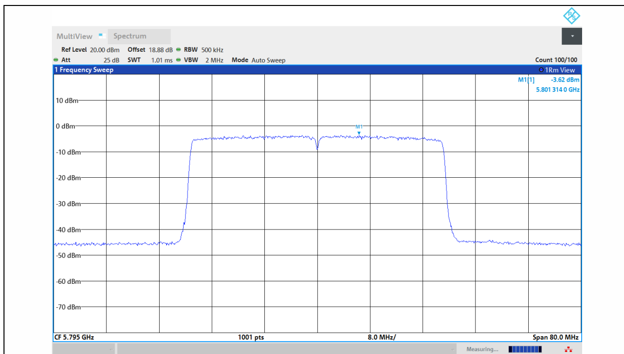
11AX40MIMO-Ant1-5795-PASS
