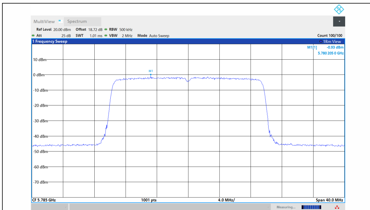
11AX20MIMO-Ant1-5785-PASS
