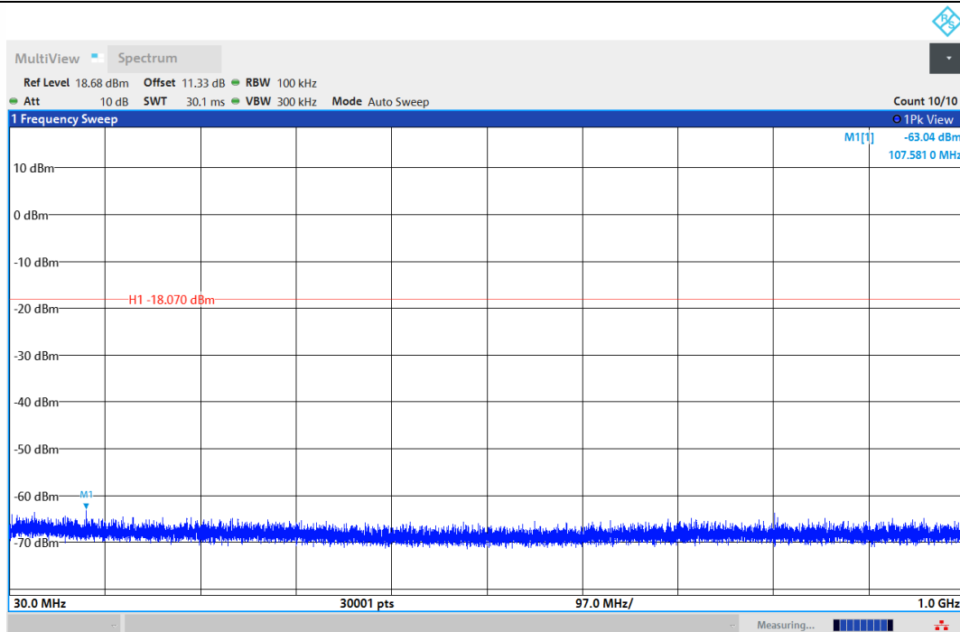
BLE_2M-Ant1-2480-30~1000-PASS
